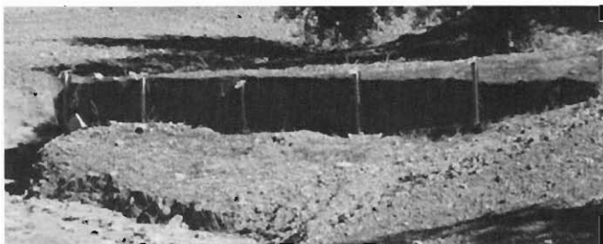
Este muro de contención ha empeorado la cárcava en vez de pararla, porque no llega bien a los dos lados de la cárcava y el agua ha encontrado como pasar por un lado de la estructura
