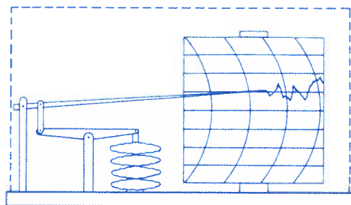
Barógrafo
