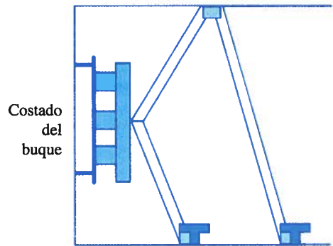
Apuntalamiento por el método triangular
