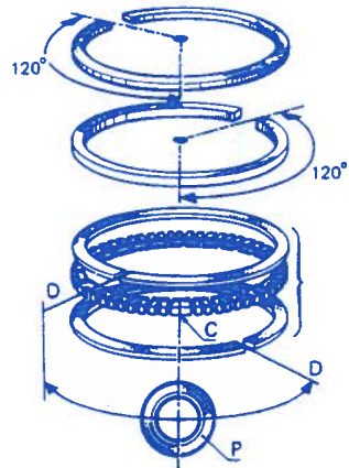
Fig. 16. Juego de aros.
