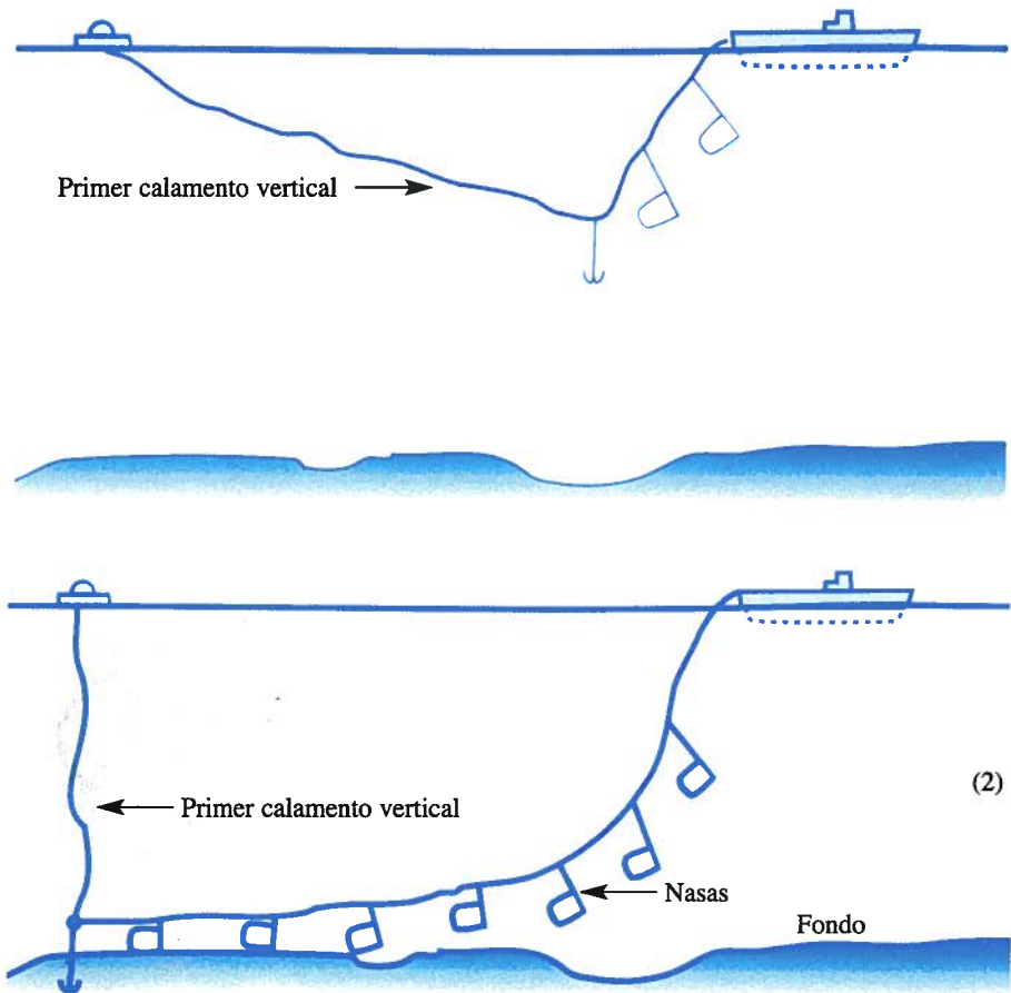
Palangre de nasas
