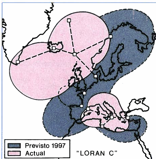
Figura 2.13. Cobertura europea del sistema "Loran C"
