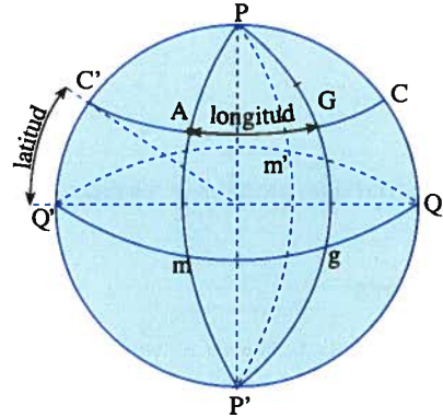
Arcos correspondientes a latitud y longitud
