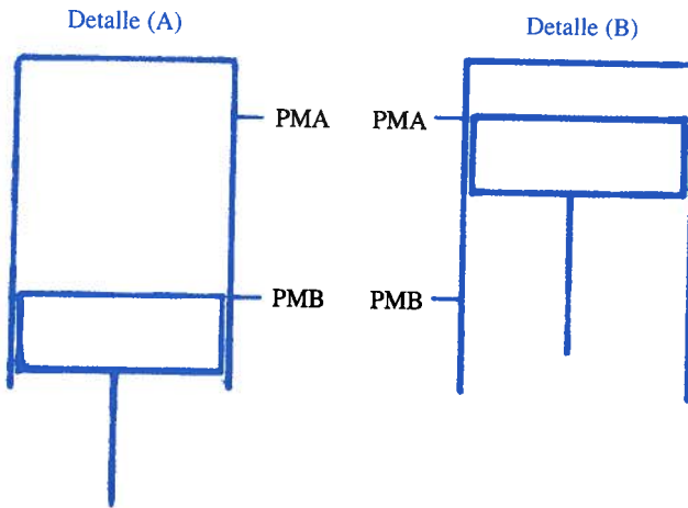
Fig. 29. Volumen total del cilindro y volumen de espacio neutro.
