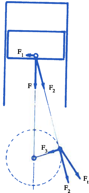
Fig. 38. La fuerza tangencial origina el movimiento del eje de cigüeñal.
