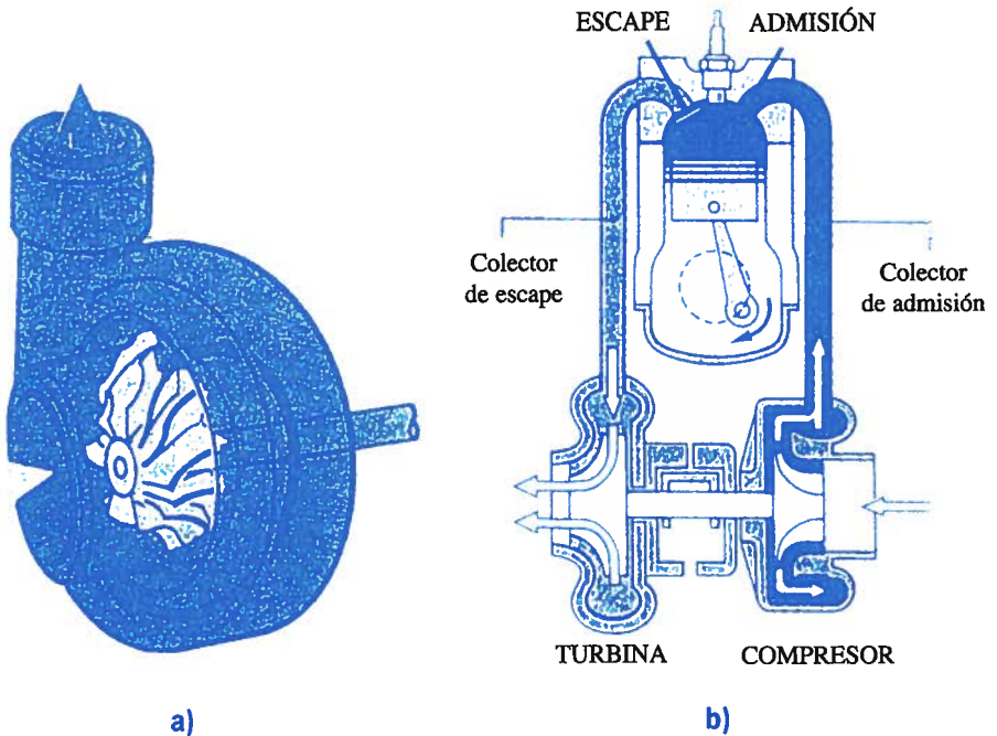
Fig. 45. a) Compresor rotativo. b) Esquema de un motor dotado de turbo-compresor
