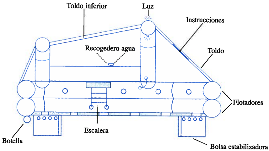
Esquema de una balsa
