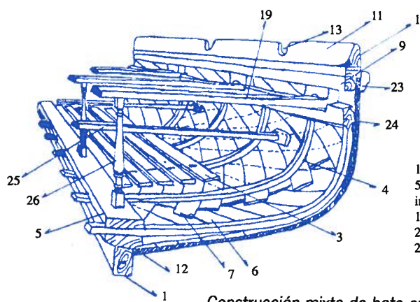
Construcción mixta de bote en madera.
