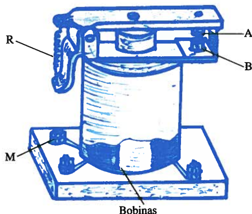
Fig. 57. Disyuntor.
