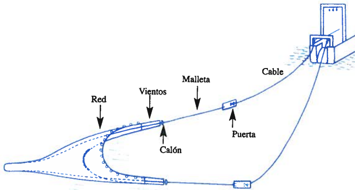
Calamento de un buque de arrastre
