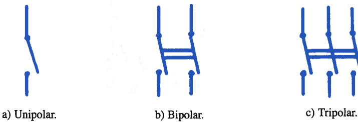
Fig. 62. Simbología de interruptores.
