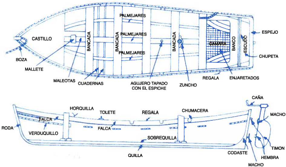
Bote y su nomenclatura
