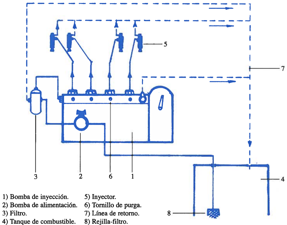
Fig. 30. Sistema de inyección combustible.
