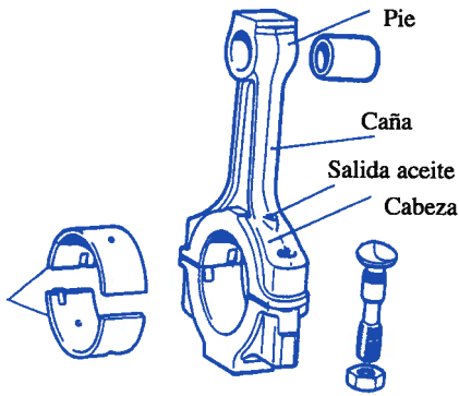
Fig. 17. Biela.
