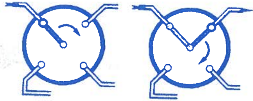
Fig. 63. Conmutador monopolar de tres circuitos
