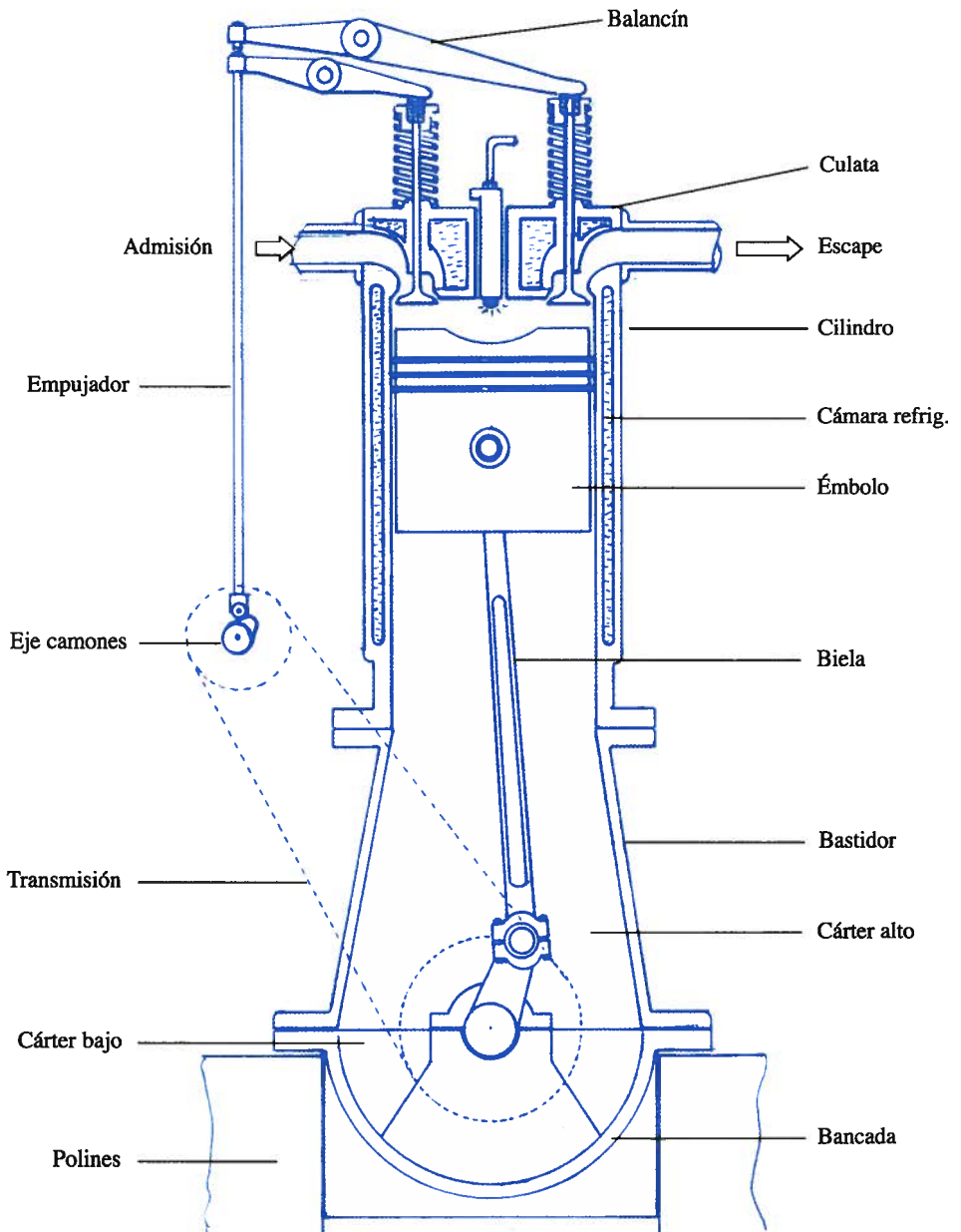
Fig. 10. Elementos de constitución de un motor.
