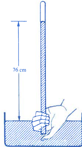
El experimento de Torricelli
