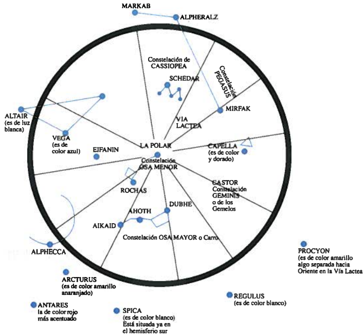
Vista del cielo con la representación de las Constelaciones Osa Menor, Osa Mayor y Cassiopea
