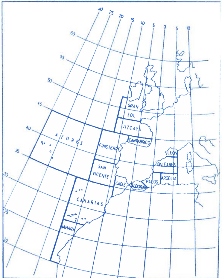
Zonas de previsión del tiempo (España). (Con autorización de la OMM)
