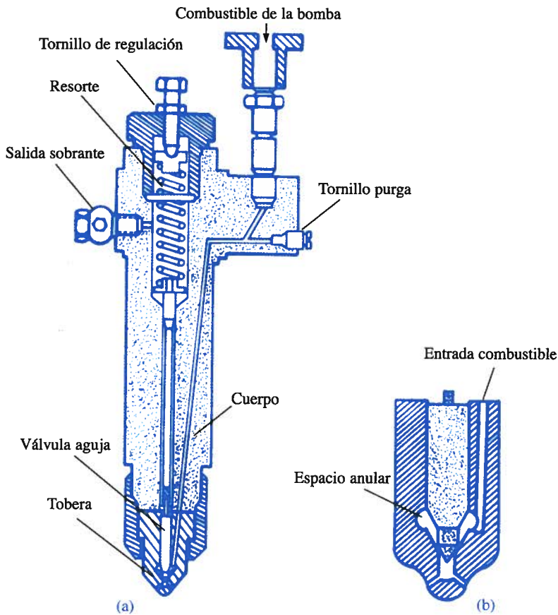
Fig. 31. a) Inyector. b) Tobera.
