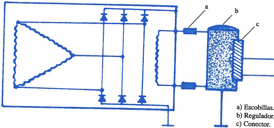
Fig. 60. Esquema eléctrico de un alternador en triángulo.
