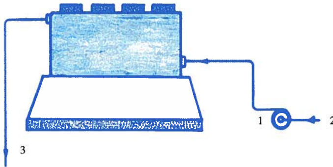
Fig. 37. Circuito abierto de refrigeración.
