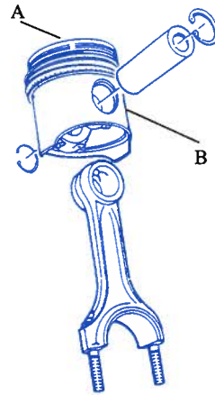
Fig. 15. Juego de pistón y biela.
