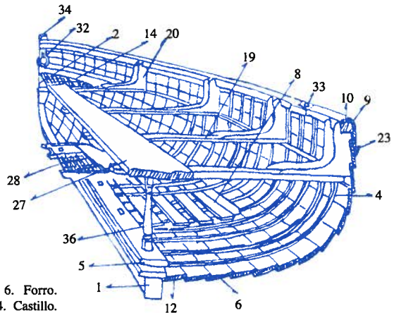
Construcción a tingladillo de bote en madera
