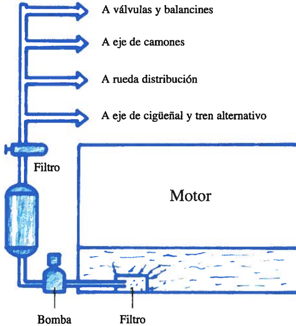
Fig. 35. Circuito esquemático de lubricación.
