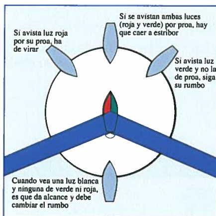
Maniobra a realizar según el tipo de luces avistadas
