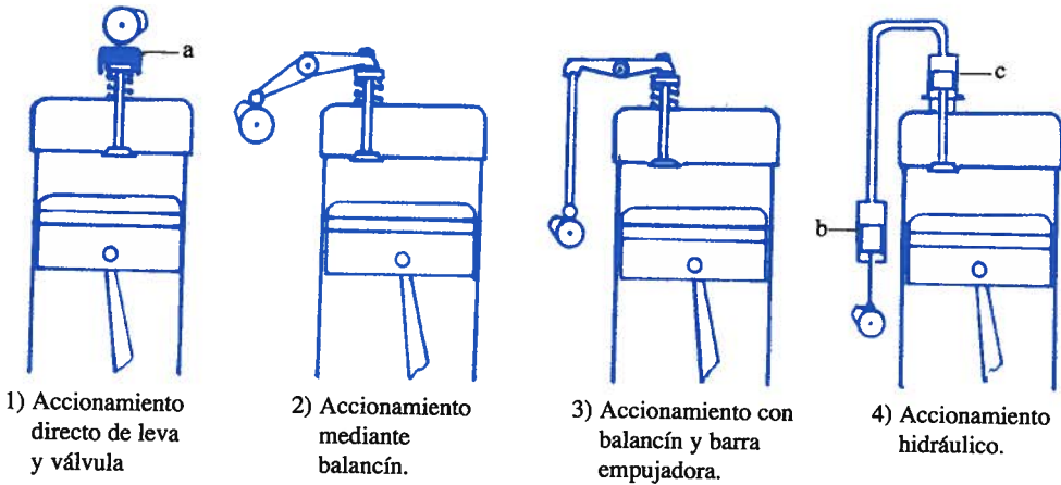
Fig. 25. Diferentes tipos de accionamientos.
