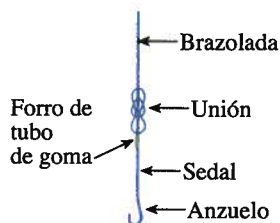
Palangre de superficie
