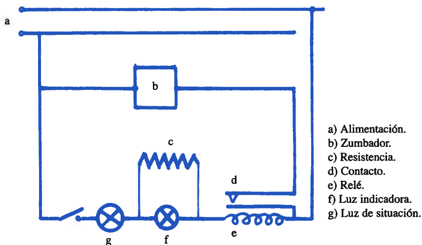
Fig. 72. Sistema de aviso de fallos de luces de navegación.
