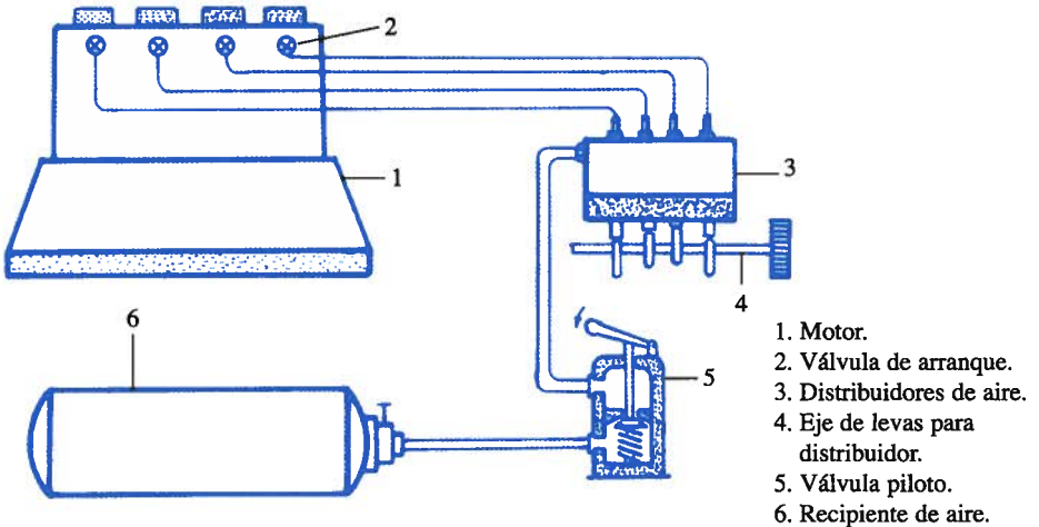
Fig. 40. Esquema simplificado del sistema de arranque por aire comprimido.
