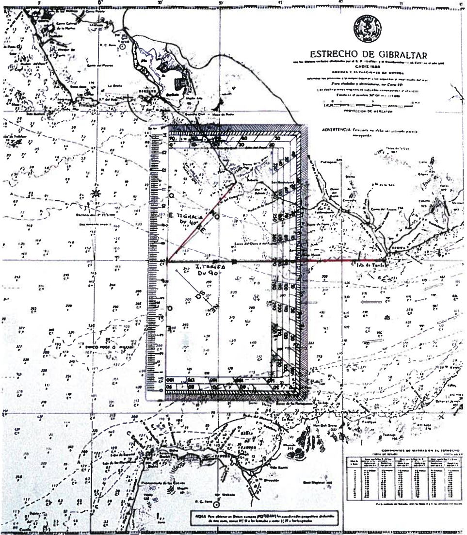
Figura 2.11. Situación por Dv a dos puntos
