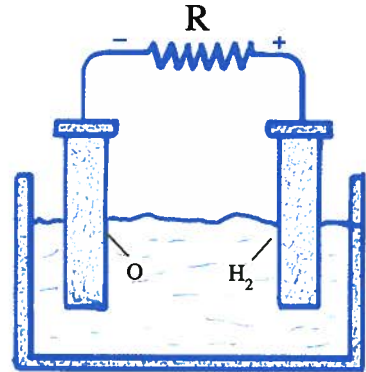
R = resistencia u otro aparato de consumo eléctrico.
