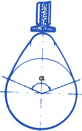
Fig. 21. Camón de perfil curvo.
