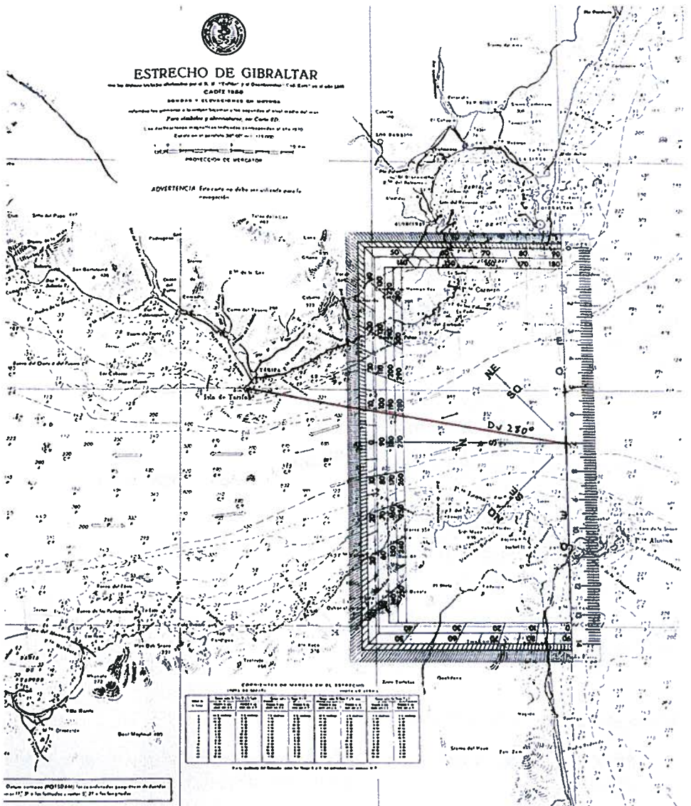
Figura 2.6. Obtención de Dv de un punto "A" desde situación estimada
