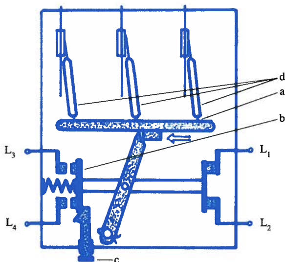
Fig. 70. Relé térmico.
