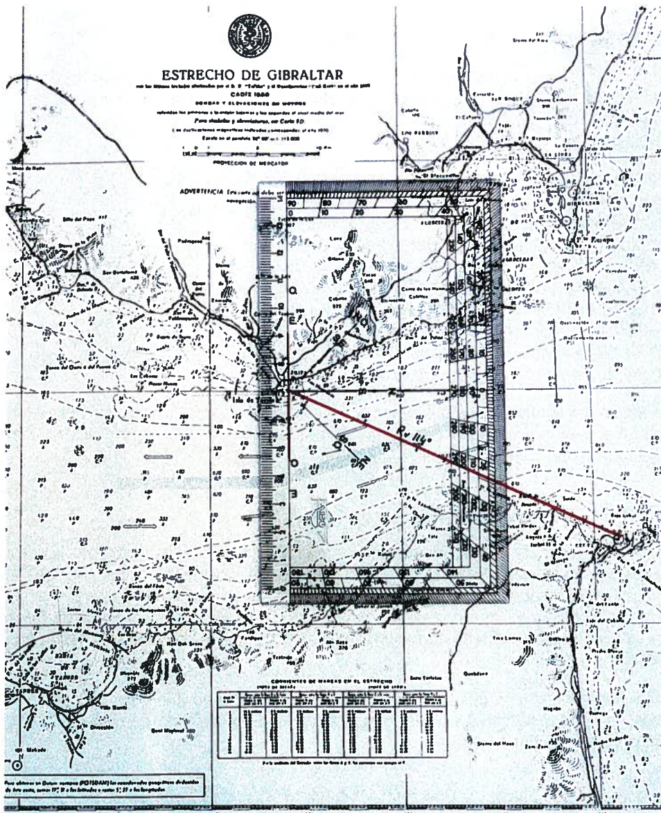
Figura 2.5. Disposición del tranportador de rumbos sobre derrota
