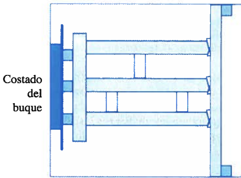
Apuntalamiento por compresión directa
