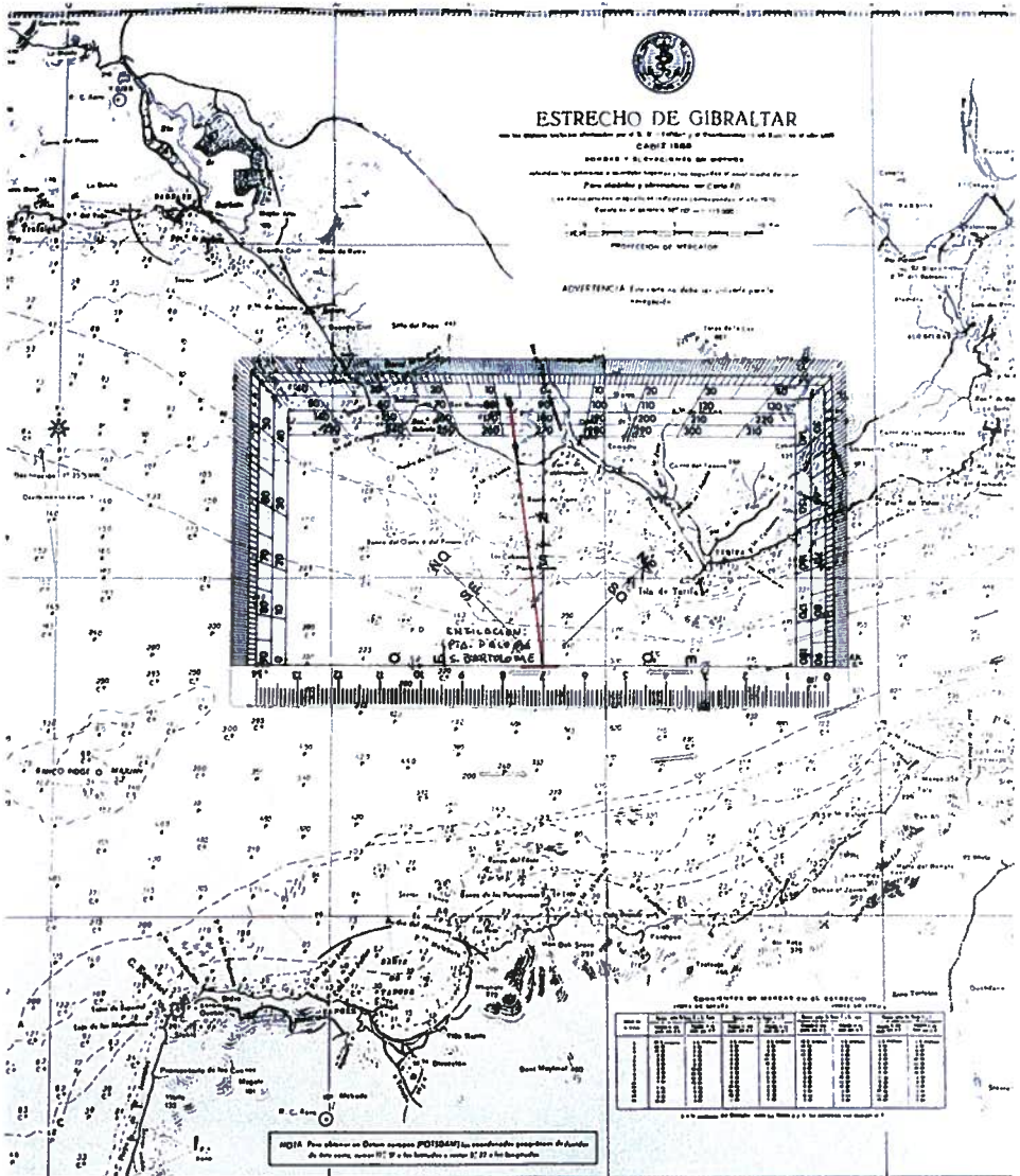
Figura 2.9. Situación por Dv de una ENFILACIÓN
