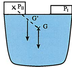
Movimiento del centro de gravedad
