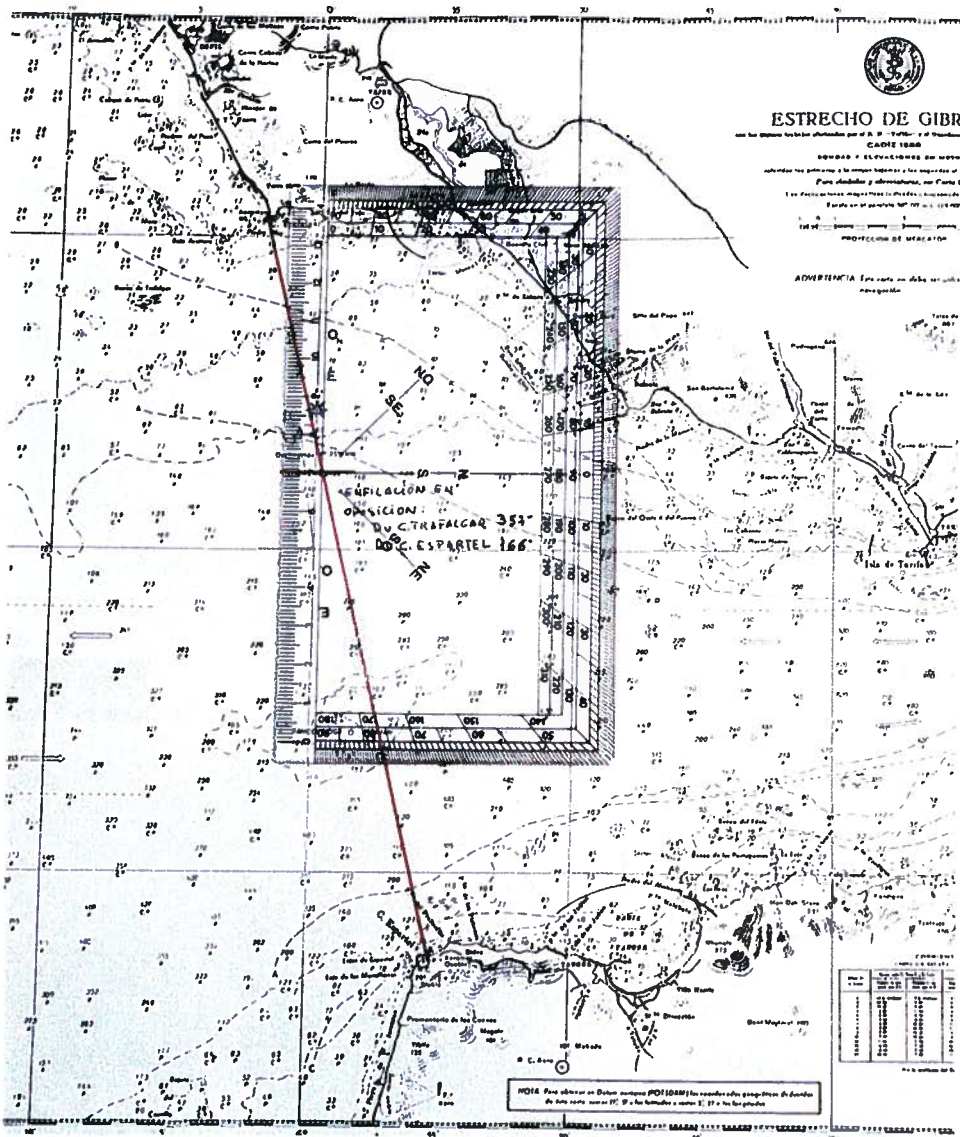
Figura 2.10. Situación por Dv a dos puntos en enfilación opuesta
