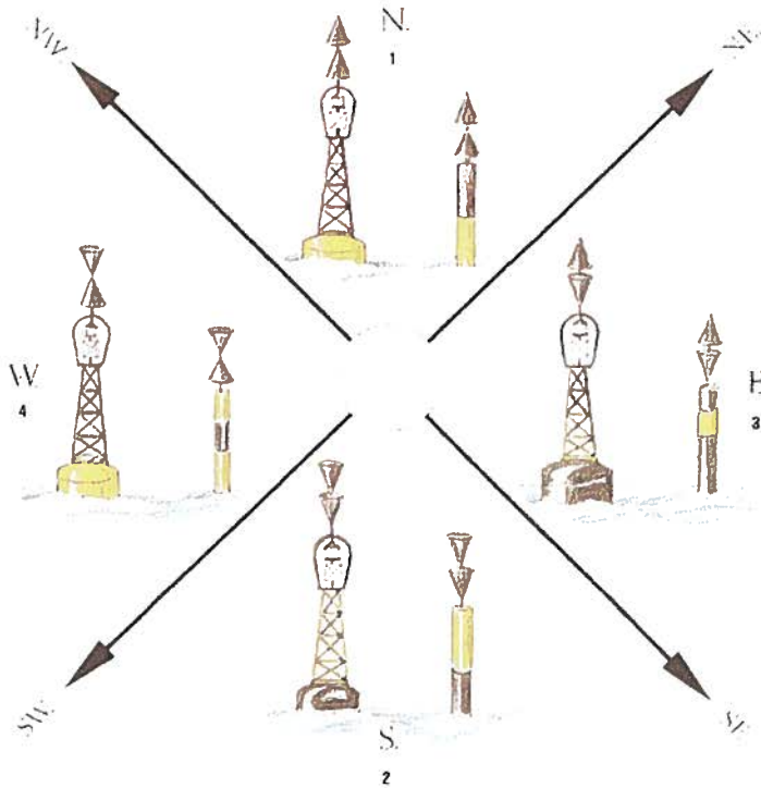
Marcas de sistema cardinal
