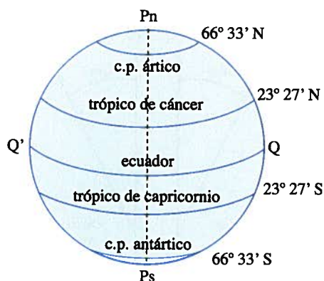
Líneas principales de la tierra
