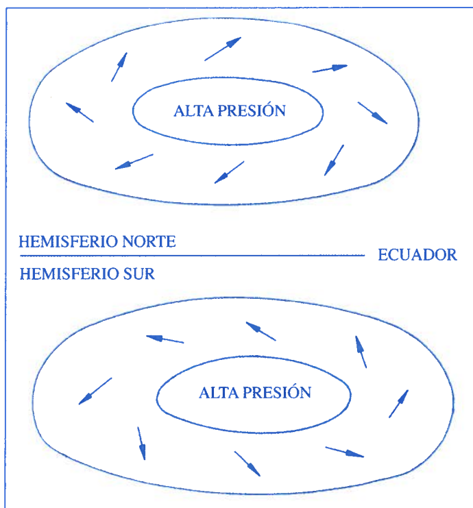
Rotación del viento alrededor de un centro de alta presión (anticiclón) en los dos hemisferios
