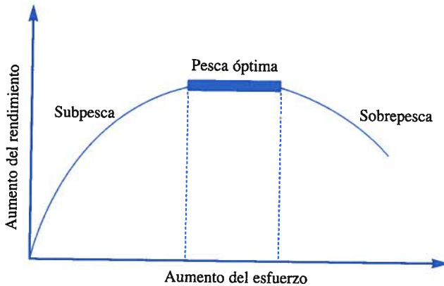
Estado de explotación de un caladero
