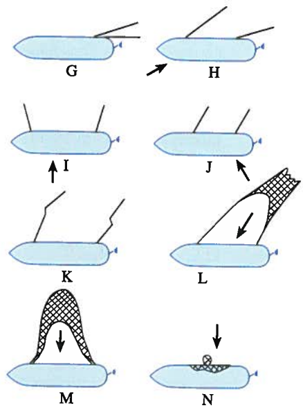
Las flechas indican el sentido del viento
