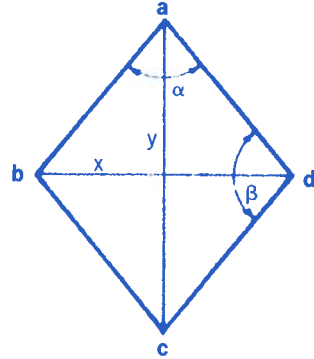
Abertura horizontal y vertical de la malla
