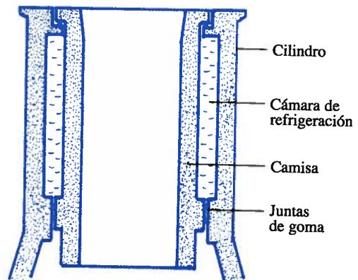
Fig. 11. Camisa postiza y húmeda.
