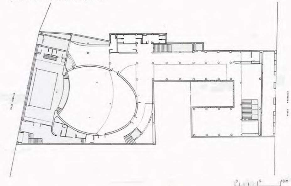
Planta Principal y Sección longitudinal
