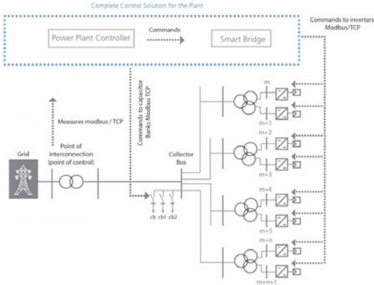
Imagen 20. Esquema sistema PPC
