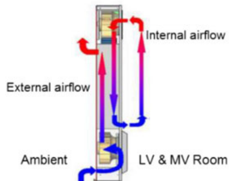
Imagen 19. Esquema de sistema de ventilación
