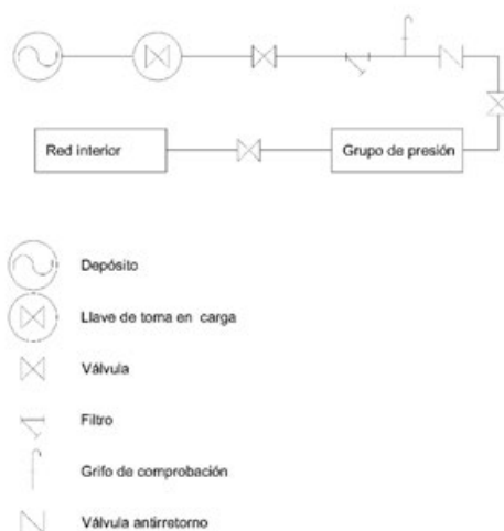
Imagen 24. Esquema instalación suministro de agua
