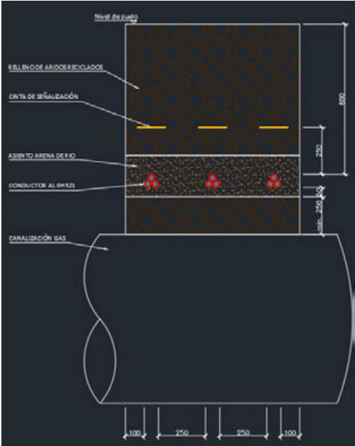
Imagen 11. Tipología de zanja empleada en el cruzamiento con gasoducto.
