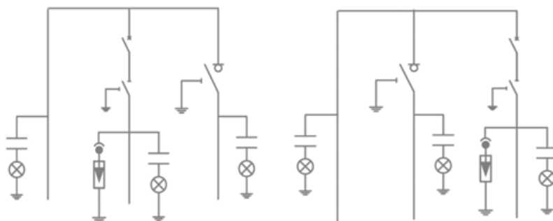
Imagen 18. Esquema de celda de MT.
