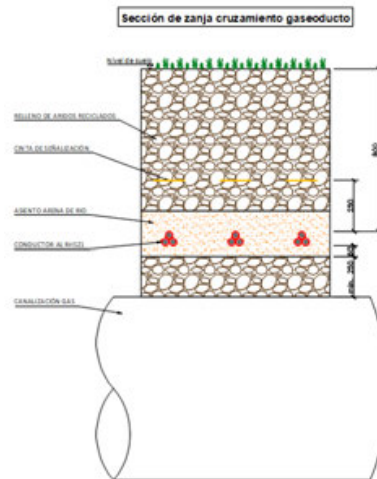
Imagen 1. Tipología de zanja empleada en el cruzamiento con gasoducto.
