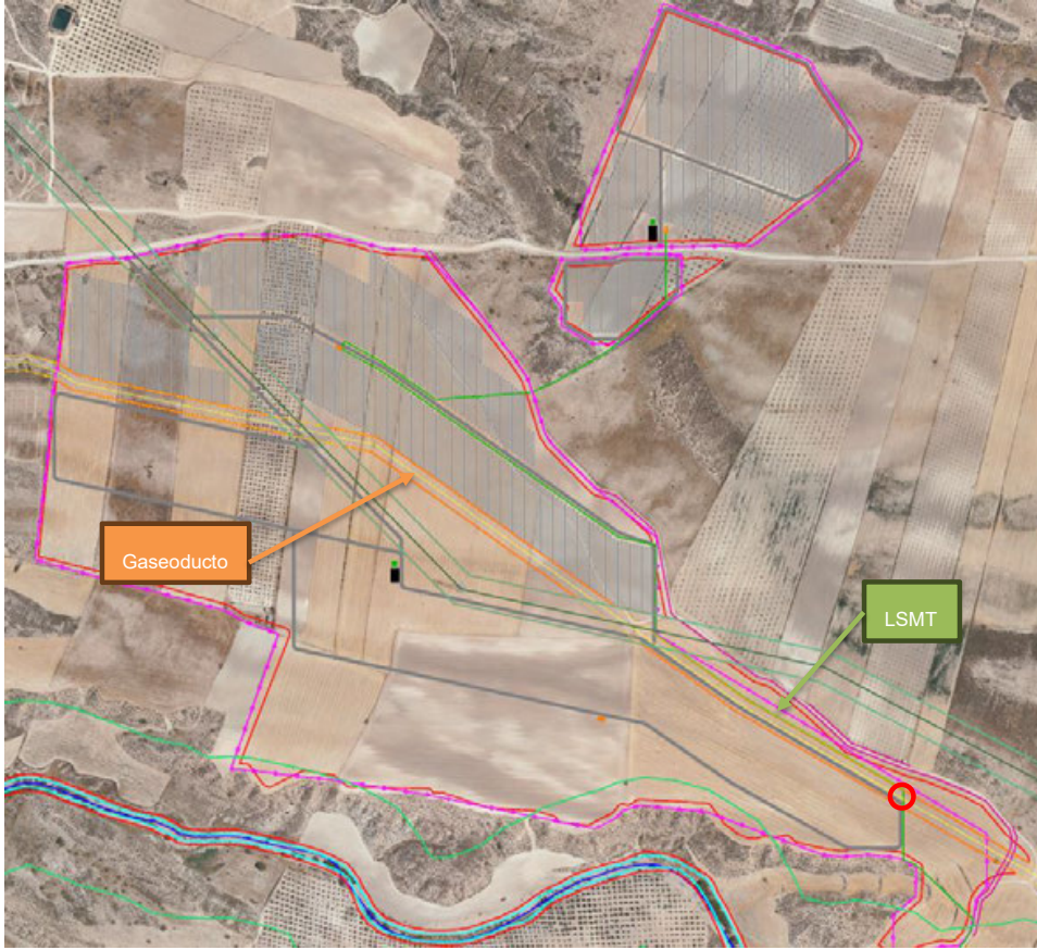
Imagen 11. Planta sobre ortofoto del primer cruzamiento con gasoducto.
