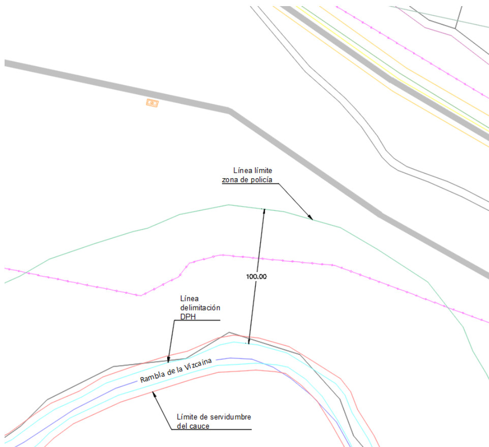
Imagen 8. Afección de la PFV Venta Angulo a la Rambla de la Vizcaína
