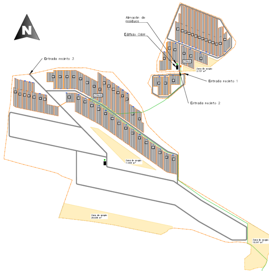
Imagen 1. Lay Out general PFV Venta Angulo
