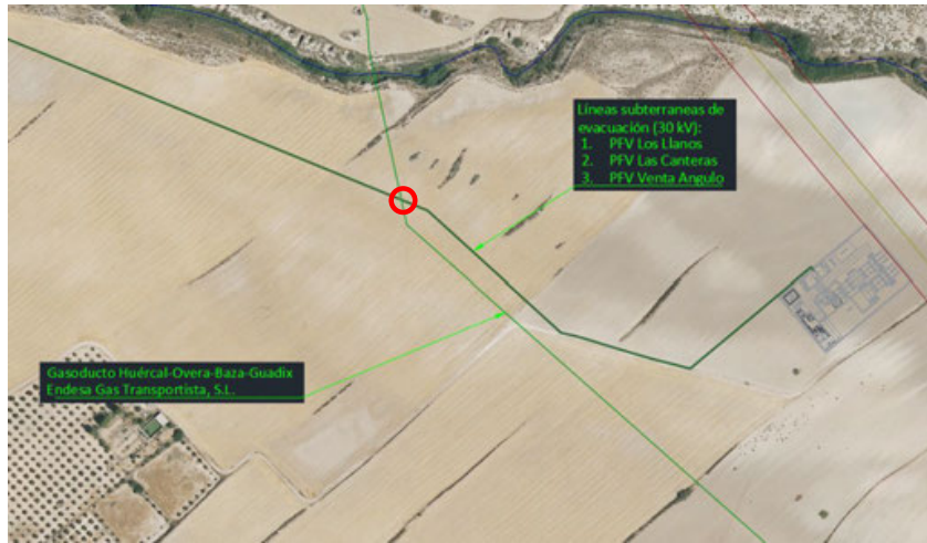
Imagen 12. Planta sobre ortofoto del segundo cruzamiento con gasoducto.
