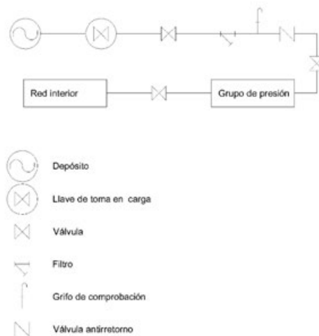
Imagen 15. Esquema instalación suministro de agua
