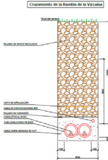
Imagen 10. Sección tipo cruzamiento con rambla
