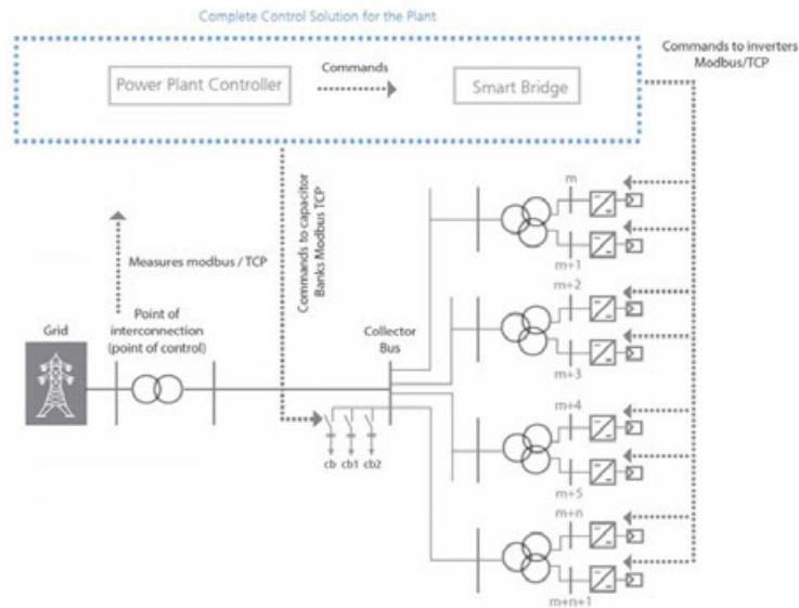
Imagen 11. Esquema sistema PPC
