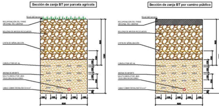
Imagen 7. Zanja tipo conexión de recintos BT
