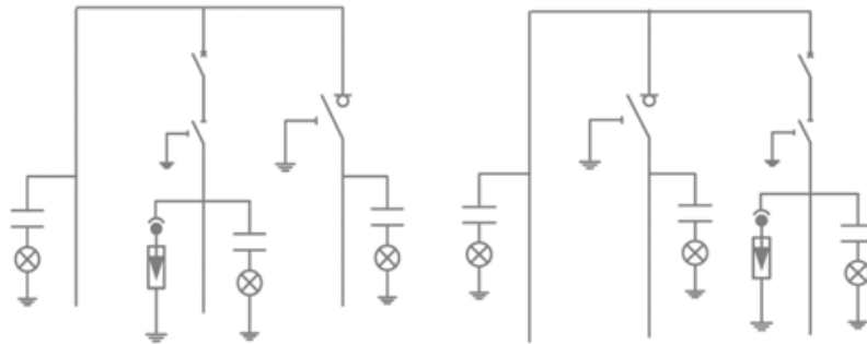
Imagen 9. Esquema de celda de MT.
