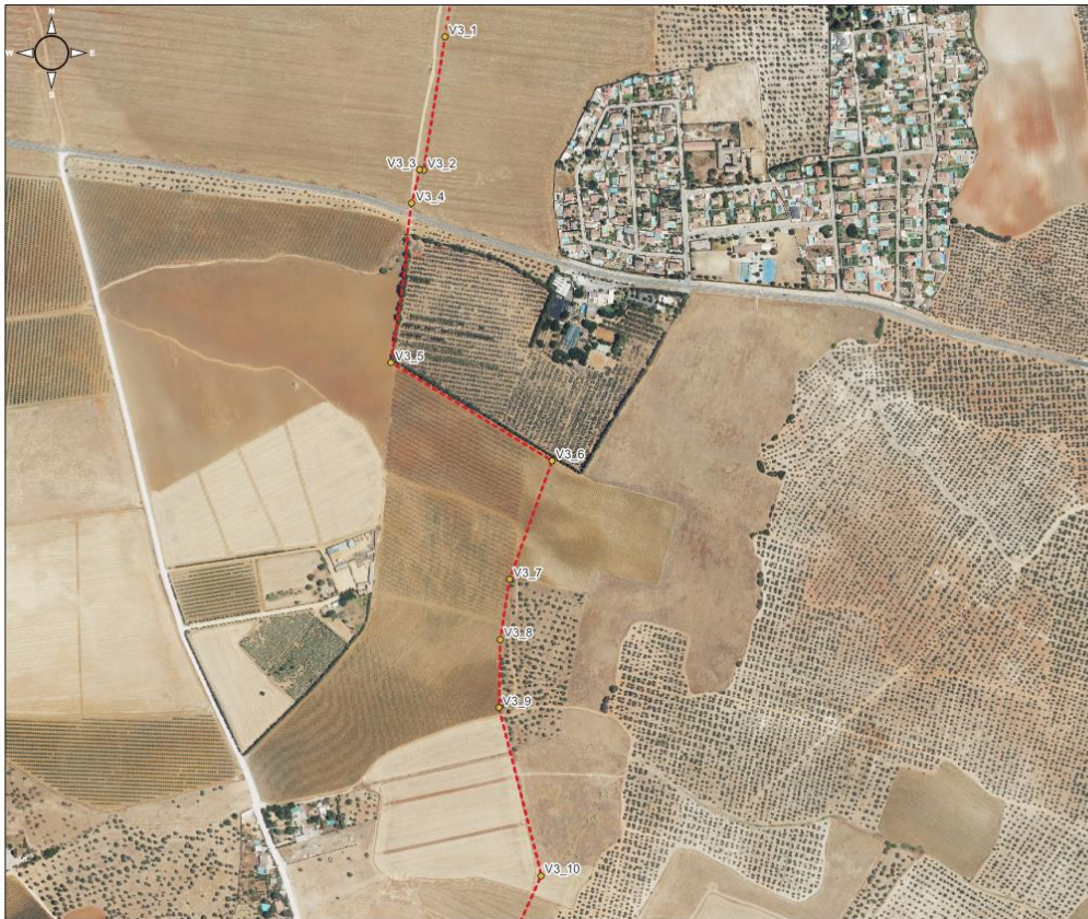
Imagen 9:Línea de evacuación subterránea 15 kV Alcalá 3 Tramo 3 (I).
