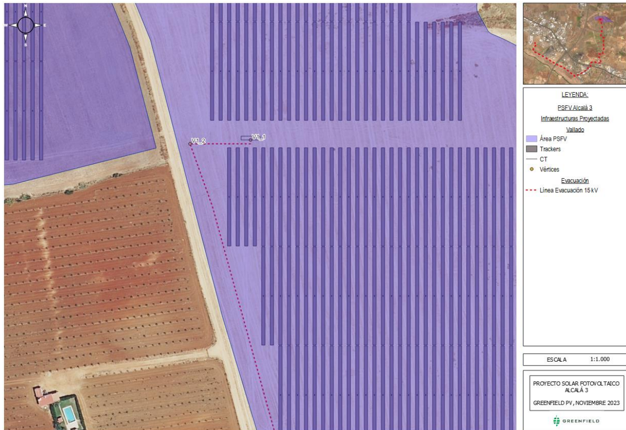
Imagen 7: Línea de evacuación subterránea 15 kV Alcalá 3 Tramo 1.
