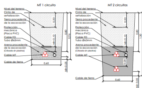
Imagen 16: Característica de la zanja interna de media tensión.
