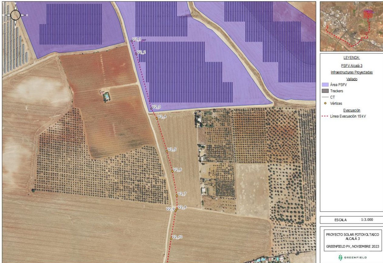
Imagen 8:Línea de evacuación subterránea 15 kV Alcalá 3 Tramo 2.
