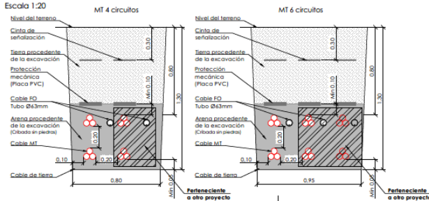
Imagen 16: Característica de la zanja interna de media tensión.
