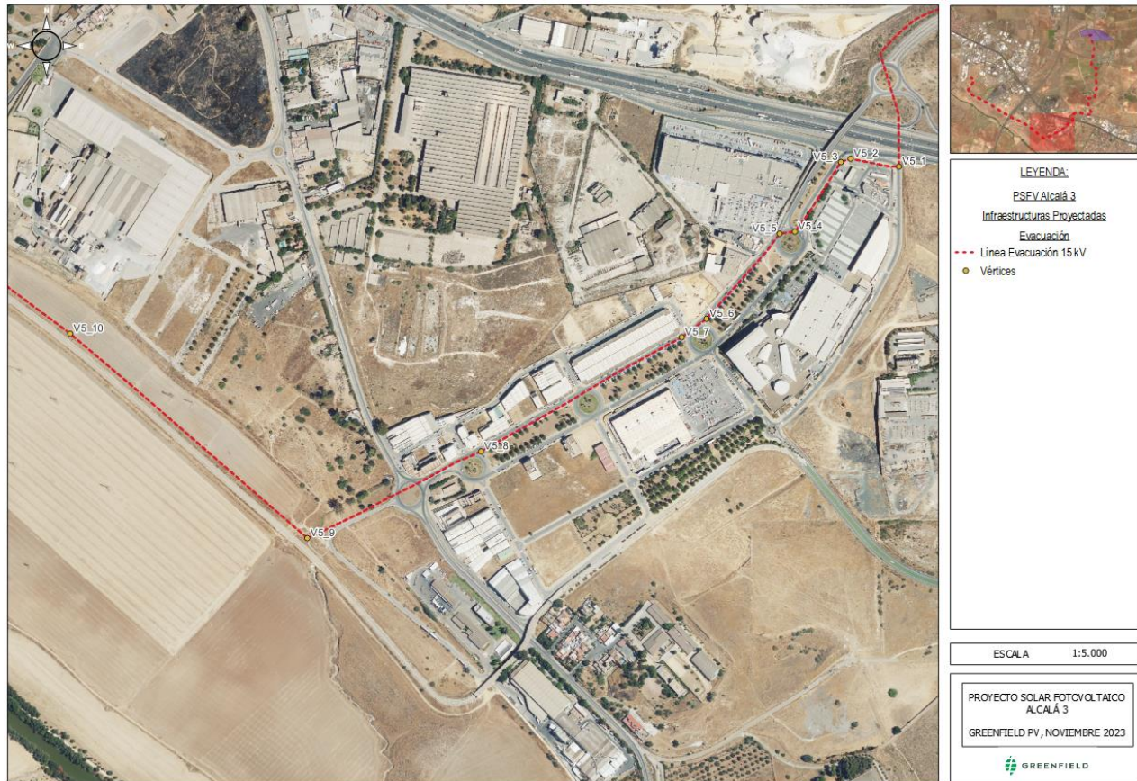
Imagen 12: Línea de evacuación subterránea 15 kV Alcalá 3 Tramo 5 (I).
