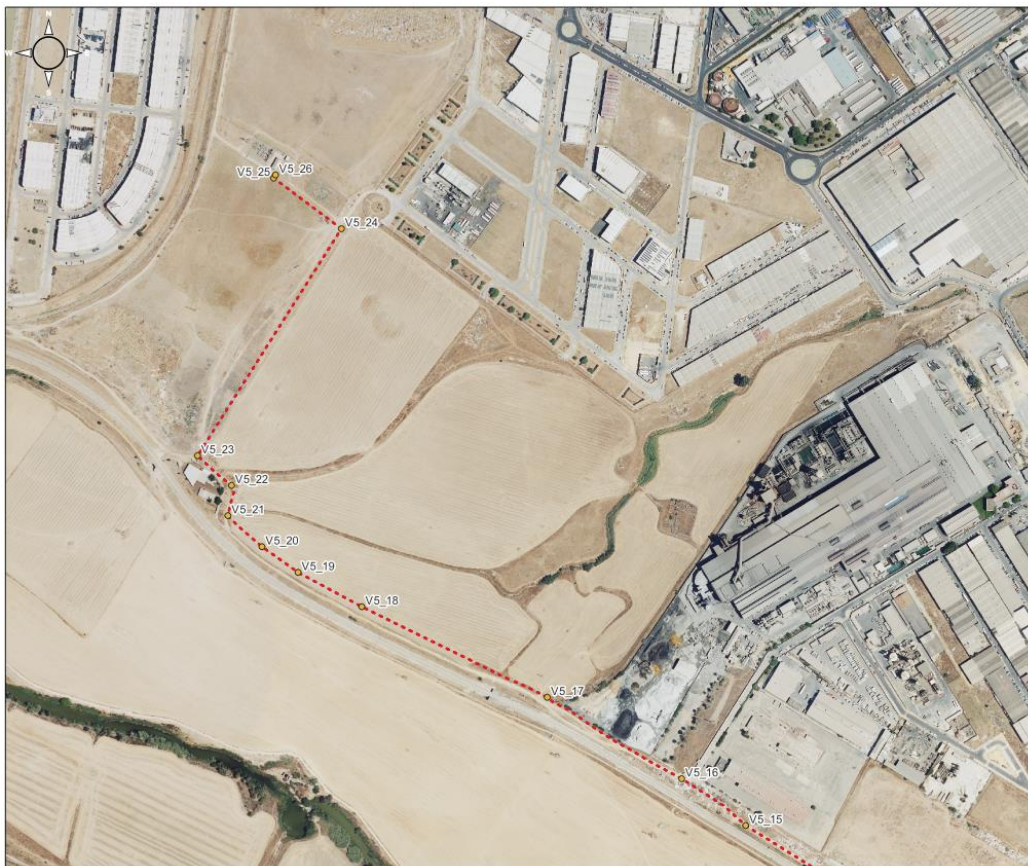
Imagen 14: Línea de evacuación subterránea 15 kV Alcalá 3 Tramo 5 (III).
