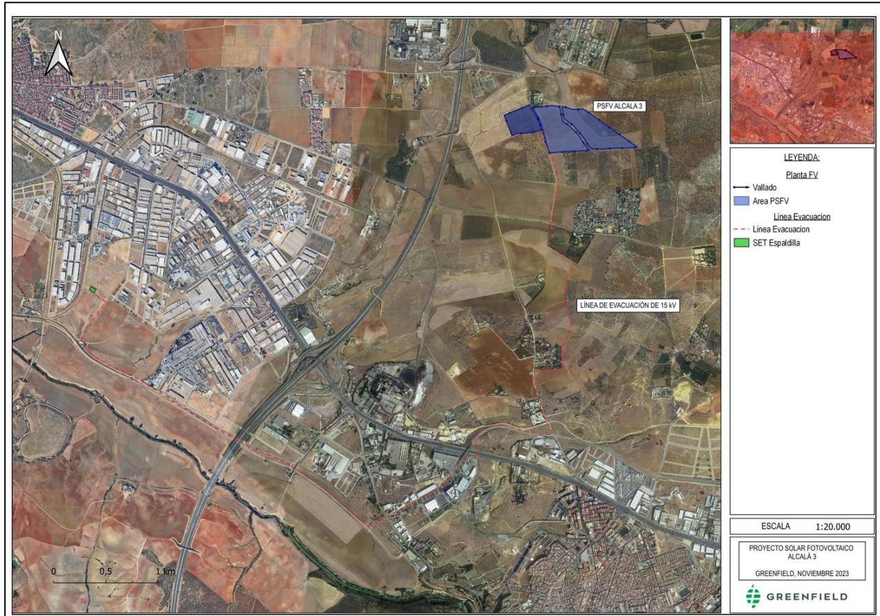
Imagen 1. Localización de la Planta Solar Fotovoltaica Alcalá 3 y Línea de Evacuación.
