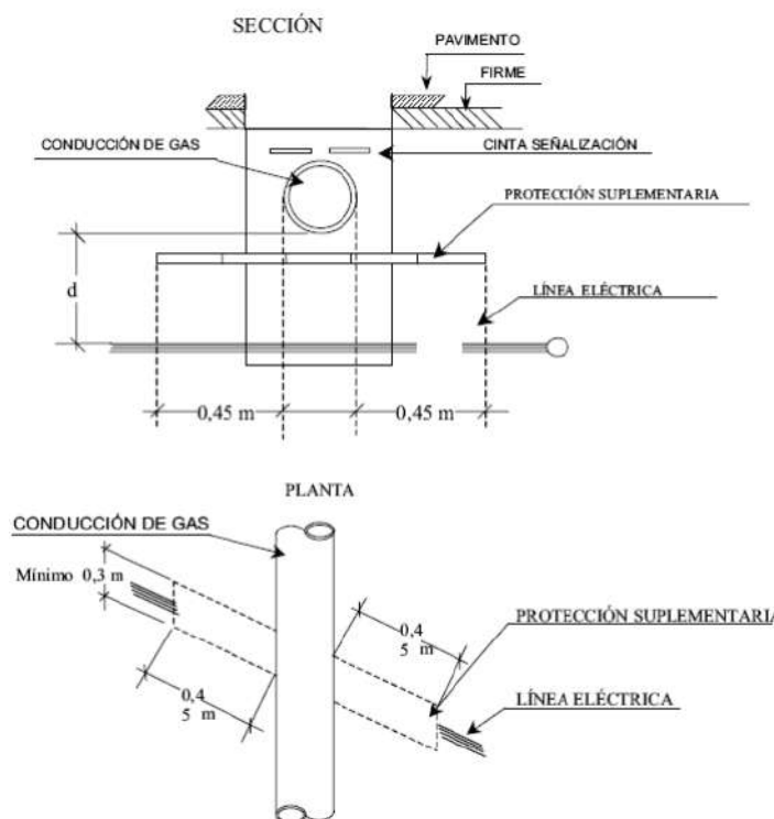
Figura 29: Detalles de cruzamiento y conducciones (ITC-LAT 06).
