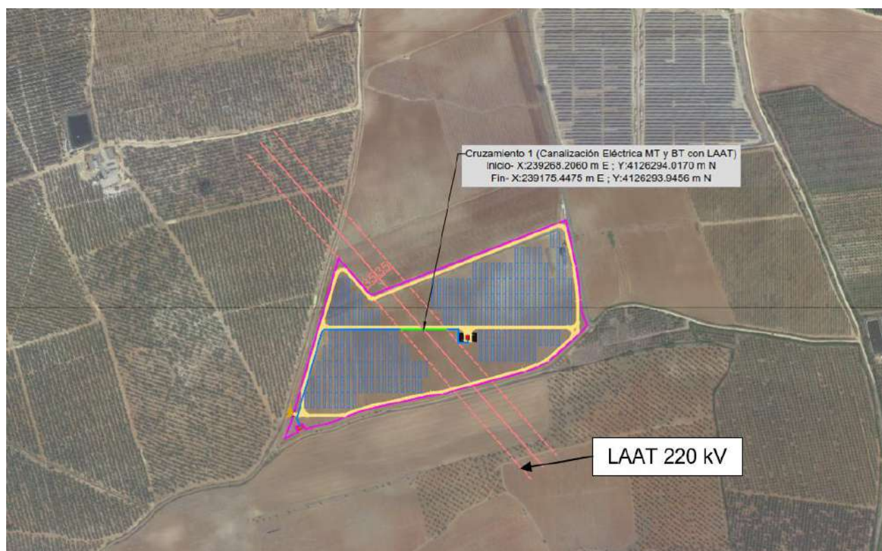
Figura 15: Localización líneas eléctricas
