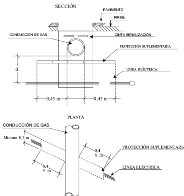
Figura 25: Detalles de cruzamiento y conducciones (ITC-LAT 06).
