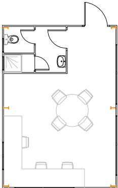
Detalle E-E' Zona Servicios Auxiliares y Oficina 1/100
