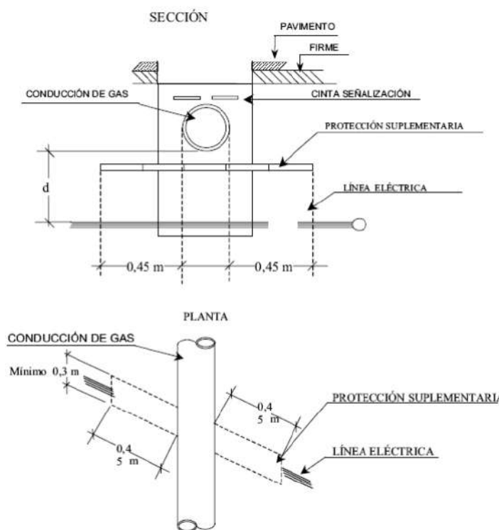
Figura 29: Detalles de cruzamiento y conducciones (ITC-LAT 06).
