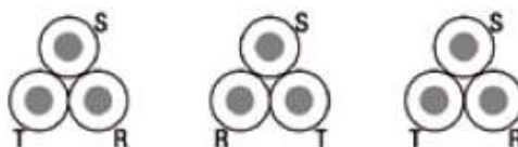
Figura 26: Colocación de cables en tresbolillo.
