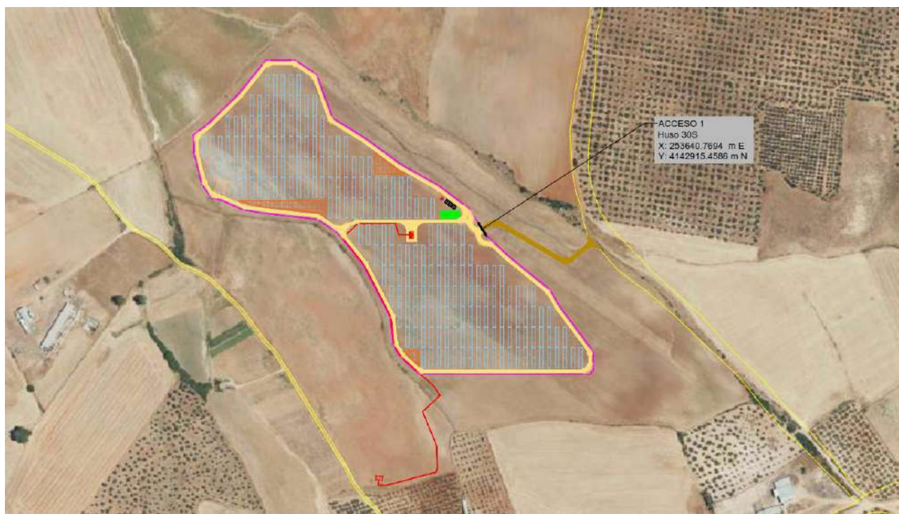
Figura 3. Accesos a la Planta Solar FV.
