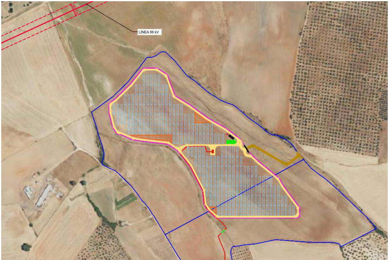
Figura 13. Líneas eléctricas
