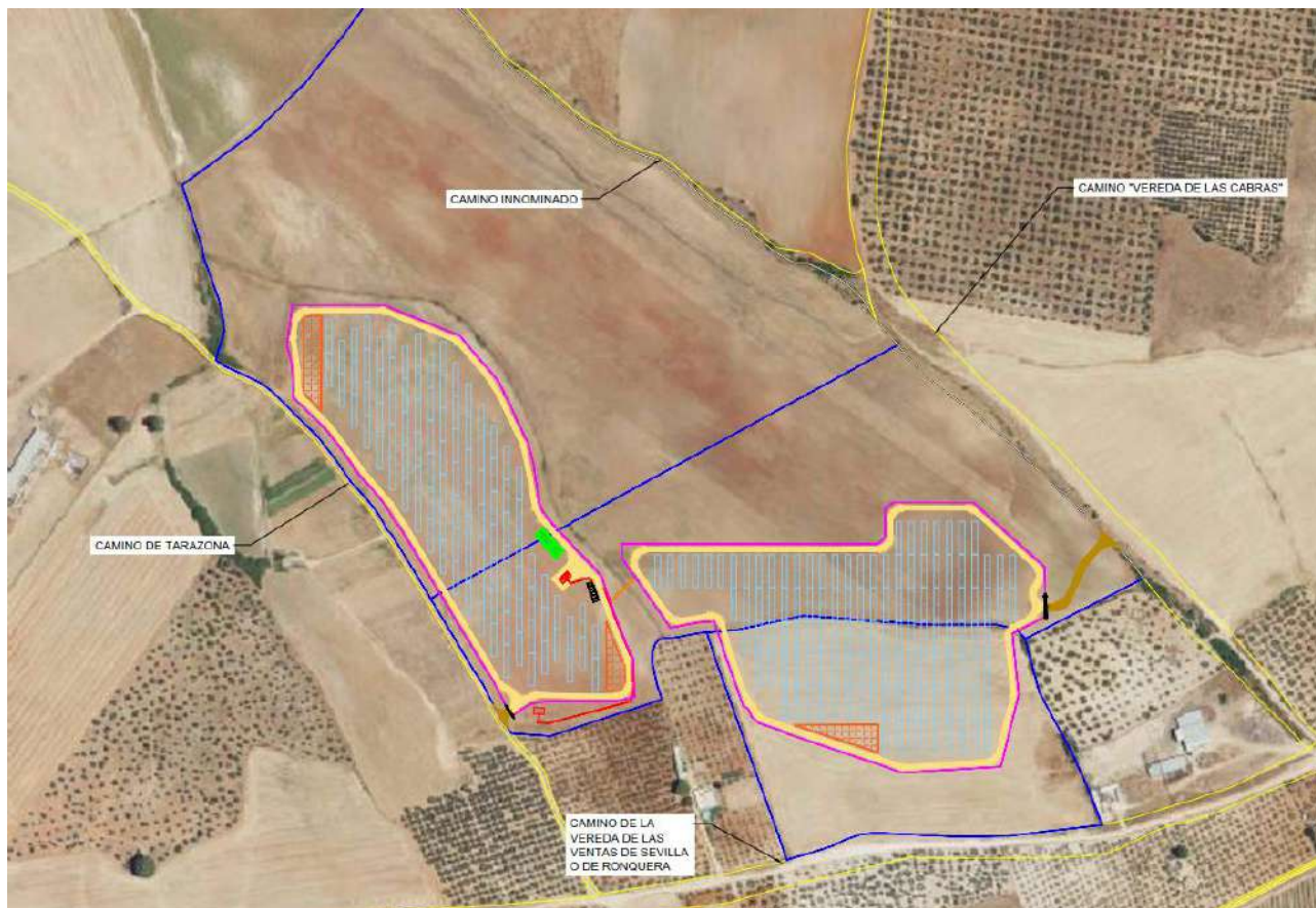
Figura 11: Caminos existentes.
