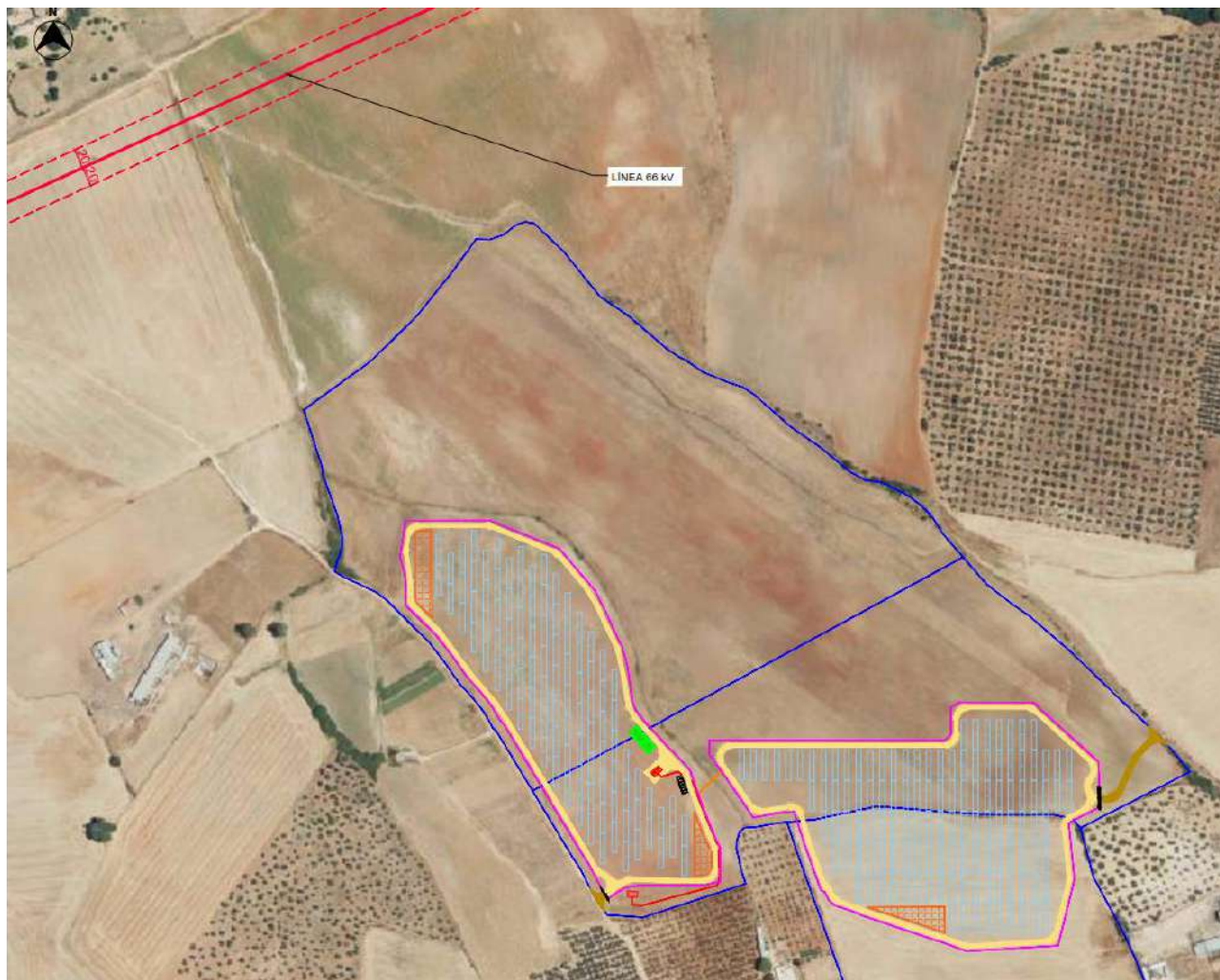
Figura 12. Líneas eléctricas existentes.
