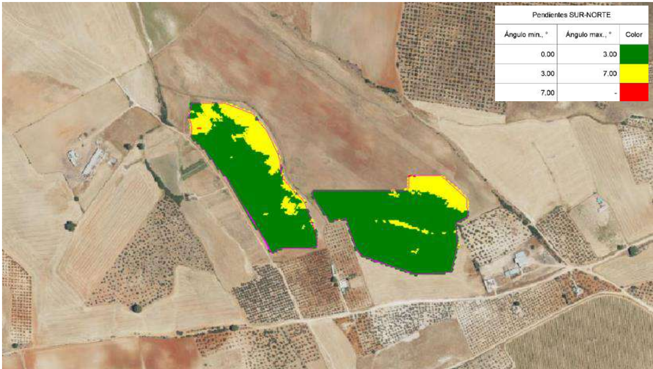
Figura 5: Pendientes S-N.
