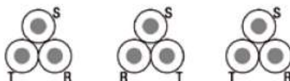
Figura 25: Colocación de cables en tresbolillo.
