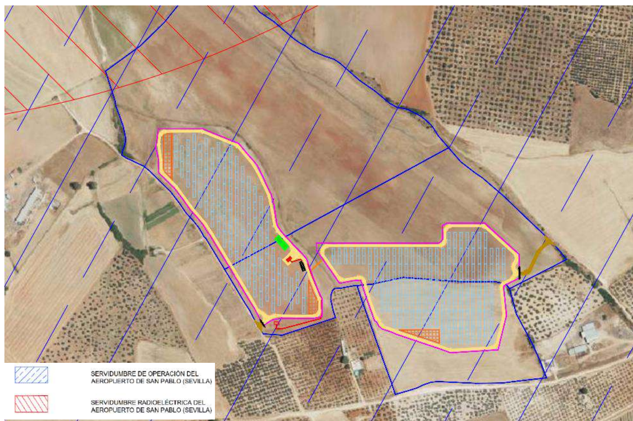
Figura 16: Servidumbre de Operación del Aeropuerto de Sevilla.
