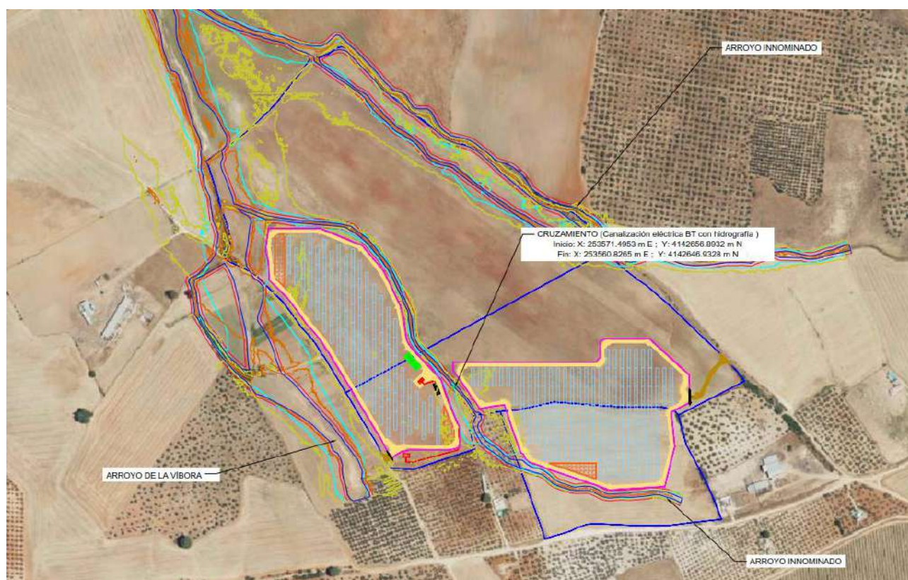
Figura 15. Red Hidrográfica Zona de Estudio.
