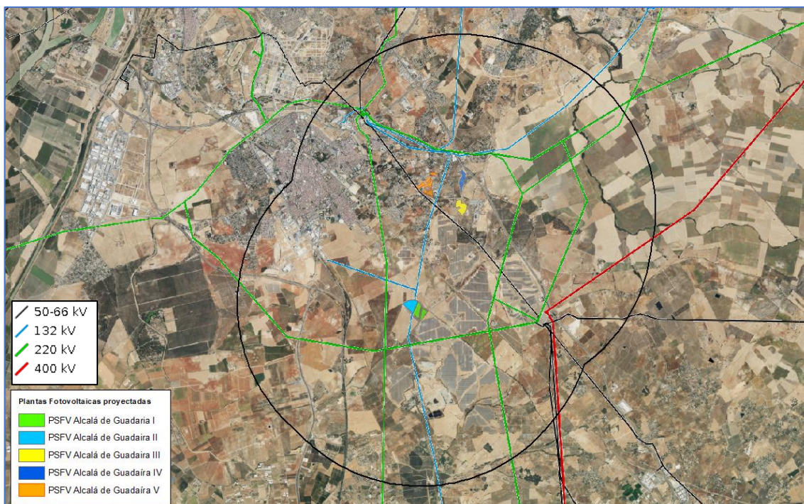
Figura 3. Infraestructuras eléctricas. Fuente: Agencia Andaluza de la Energía.
