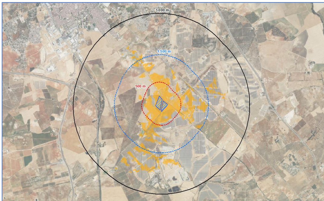
Figura 36. Visibilidad de la Planta Fotovoltaica. Elaboración propia.
