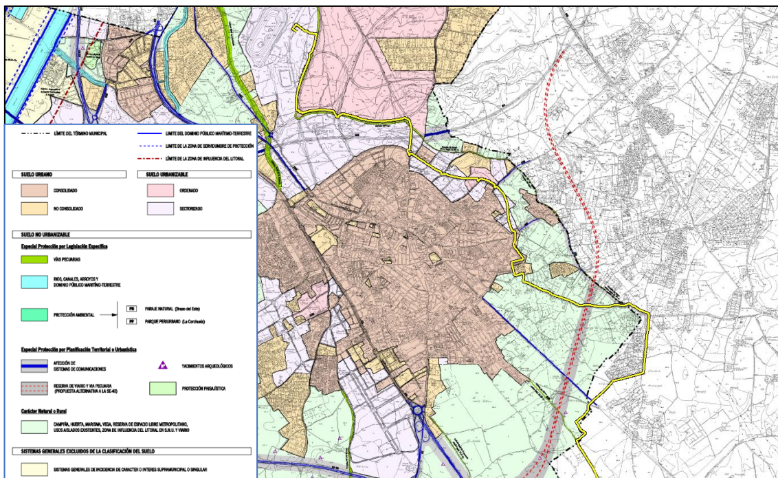
Figura 51. Representación de la línea subterránea de evacuación sobre el PGOU de Dos Hermanas. Fuente: PGOU Dos Hermanas.
