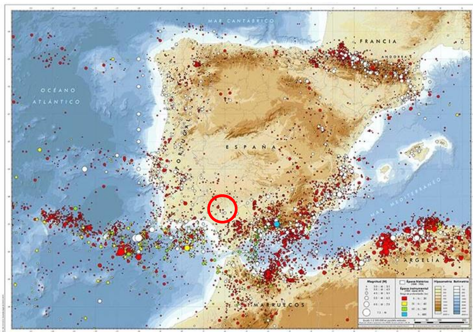
Figura 55. Sismicidad en la península ibérica y zonas próximas. Fuente: Instituto Geográfico Nacional (IGN)
