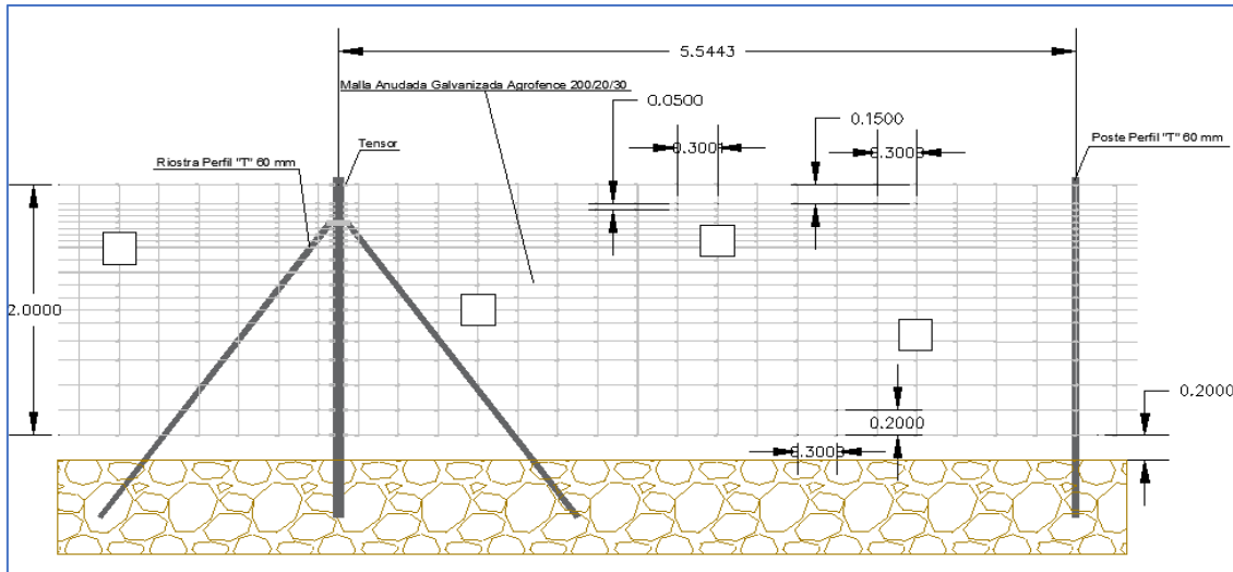
Figura 10. Vallado cinético. (Fuente: Propia)
