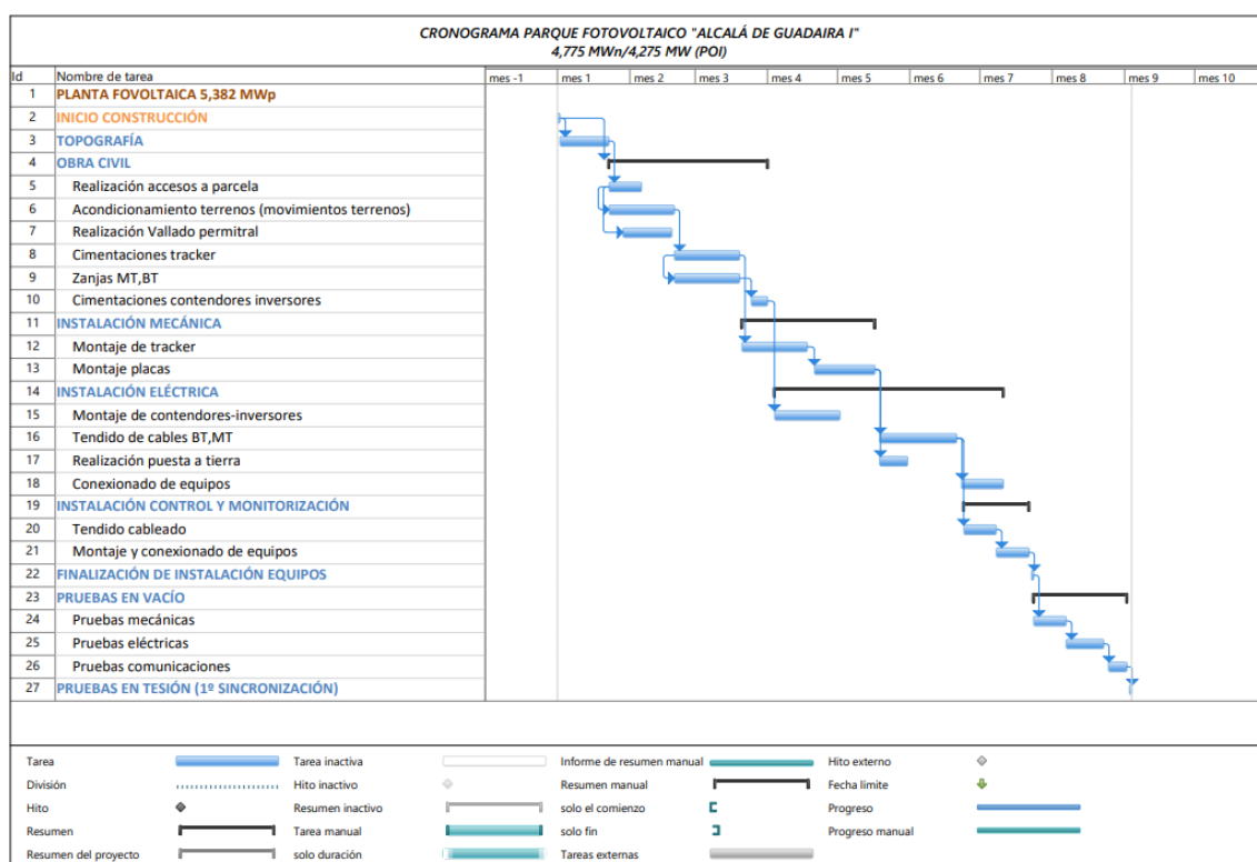
Figura 11. Cronograma de la fase de Construcción de la PSFV. Fuente: propia
