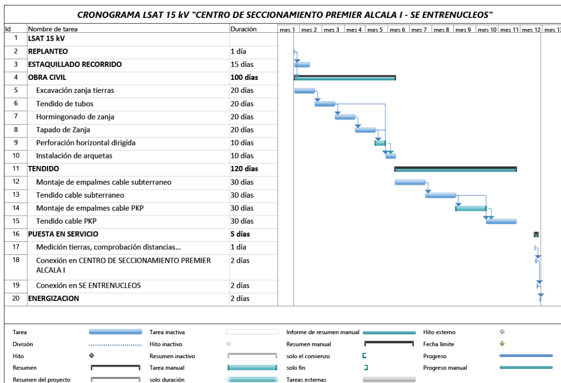
Figura 12. Cronograma de la fase de Construcción de la LSAT. Fuente: propia
