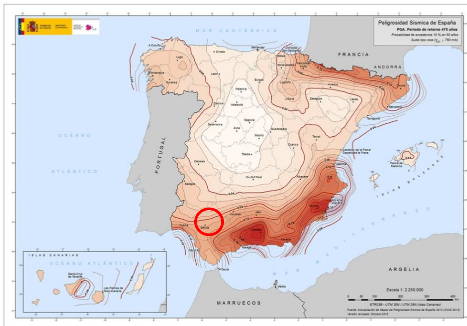
Figura 56. Peligrosidad Sísmica en España. Fuente: Instituto Geográfico Nacional (IGN)
