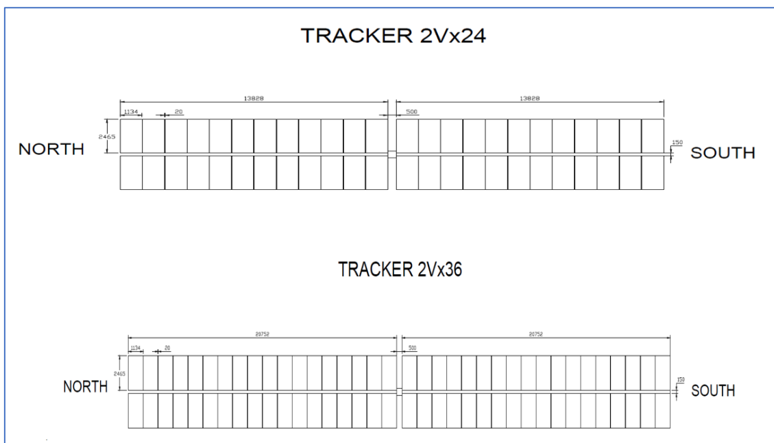
Figura 9. Tipos de configuraciones de las mesas (Fuente: Propia)
