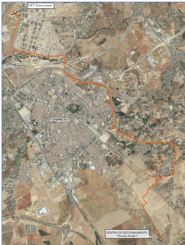
Figura 2. Infraestructuras proyectadas hasta la SET "Entrenúcleos".
