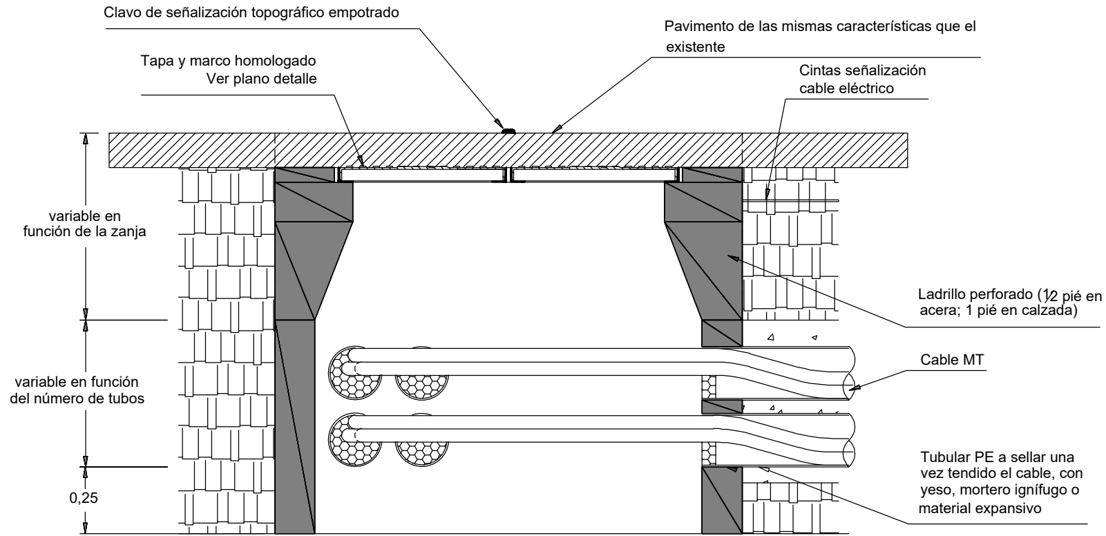
SECCIÓN A-A'
