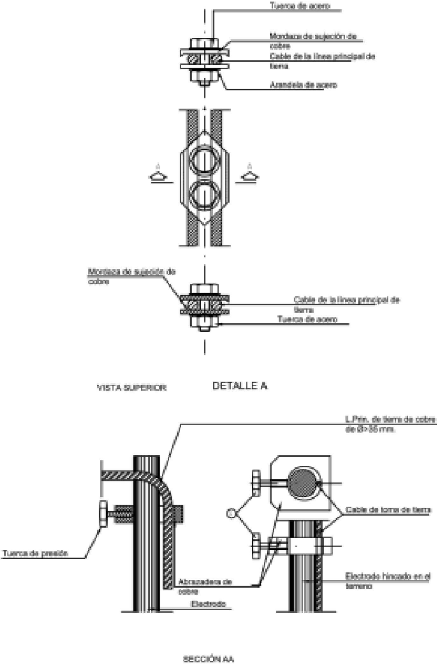
DETALLE EMPALMES LÍNEAS PRINCIPALES TOMA TIERRA
