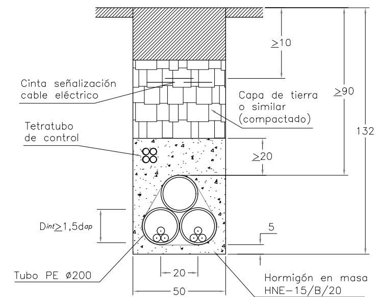
(EN CALZADA TUBO HORMIGONADO) CRUCE
