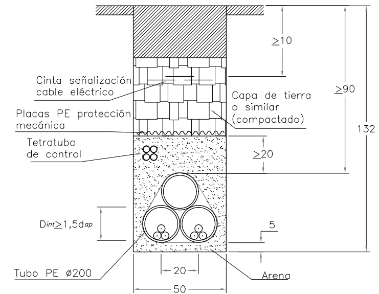
(EN CALZADA TUBO SECO)
