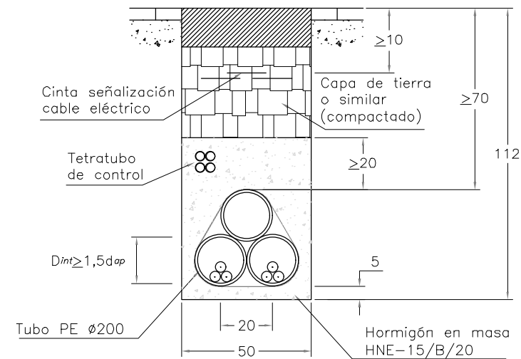
(EN ACERA TUBO HORMIGONADO)
