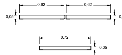
SECCIÓN MARCO A-2
