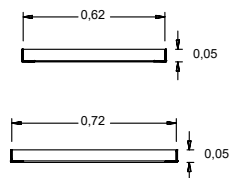
SECCIÓN MARCO A-1
