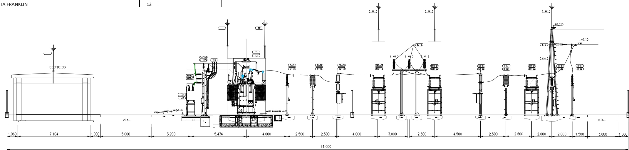
ALZADO AA
