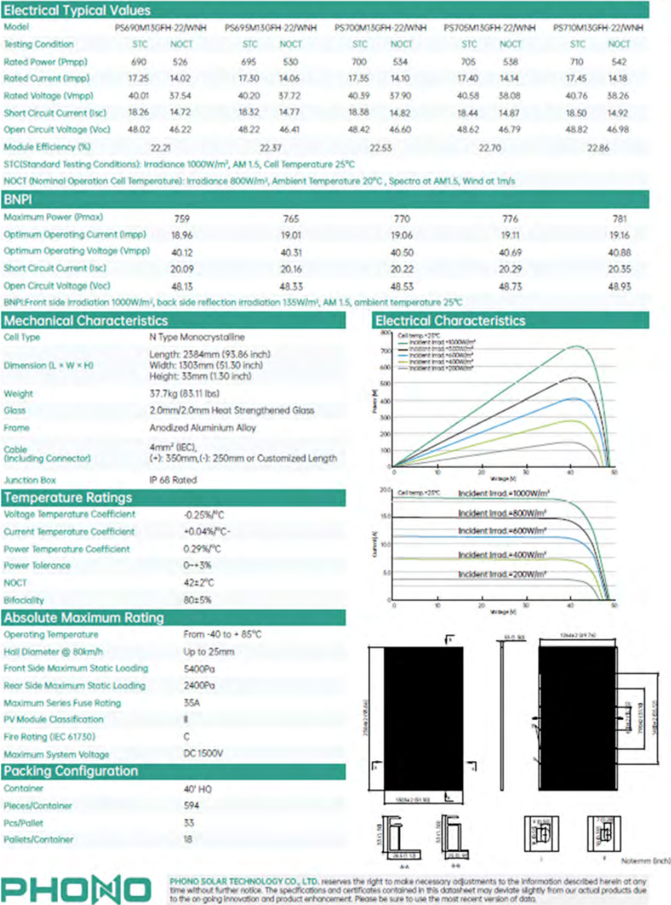
Ilustración 2: Ficha técnica módulo fotovoltaico
