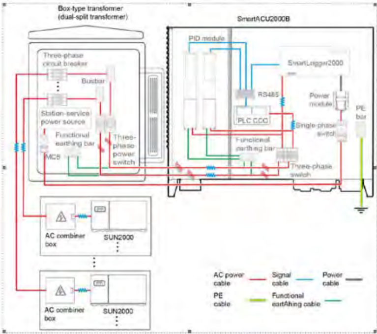
Ilustración 8: Módulo anti-PID
