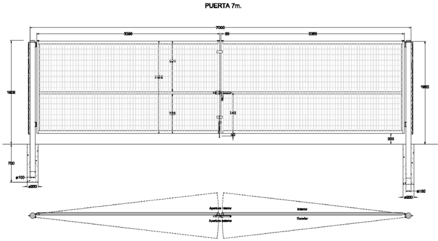
Ilustración 15: Plano de la puerta de acceso.
