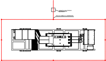
STATCOM
