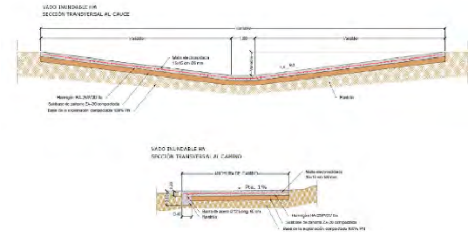
Ilustración 12: Acondicionamiento de vado existente.
