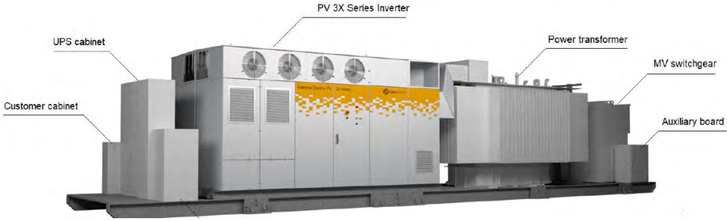
Ilustración 5: La configuración del PV Station
