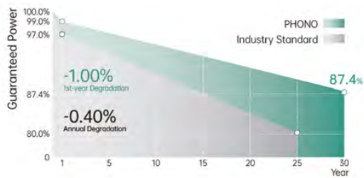
Ilustración 1: Garantía de rendimiento
