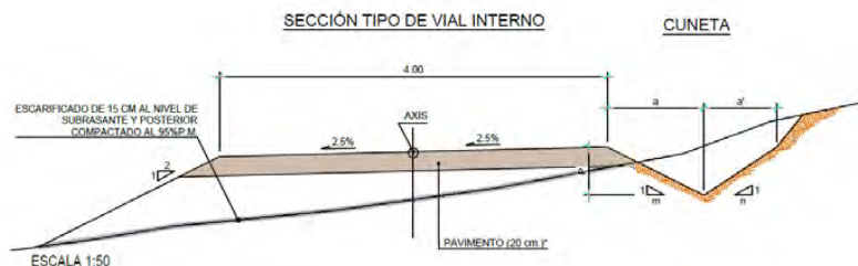
Ilustración 13: Sección tipo de vial interno.
