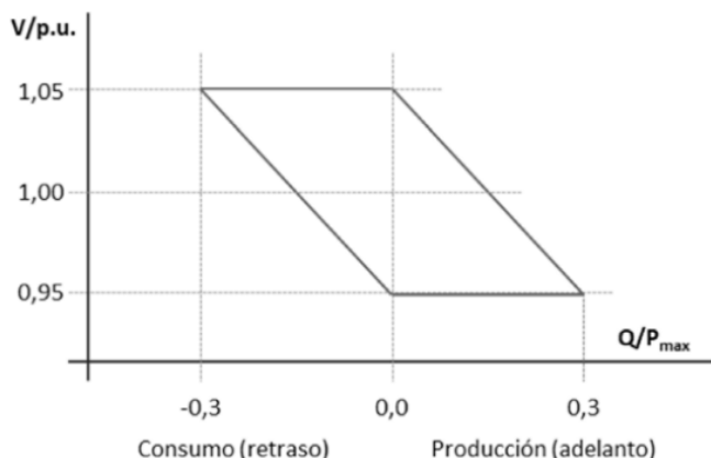
Ilustración 8: Diagrama U-Q/P de un módulo de generación de electricidad síncrono tipo C cuando P_{max} < 15 MW.
