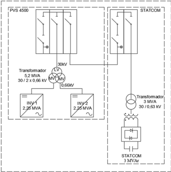
CONFIGURACIÓN CIRCUITOS DE MEDIA TENSIÓN:
