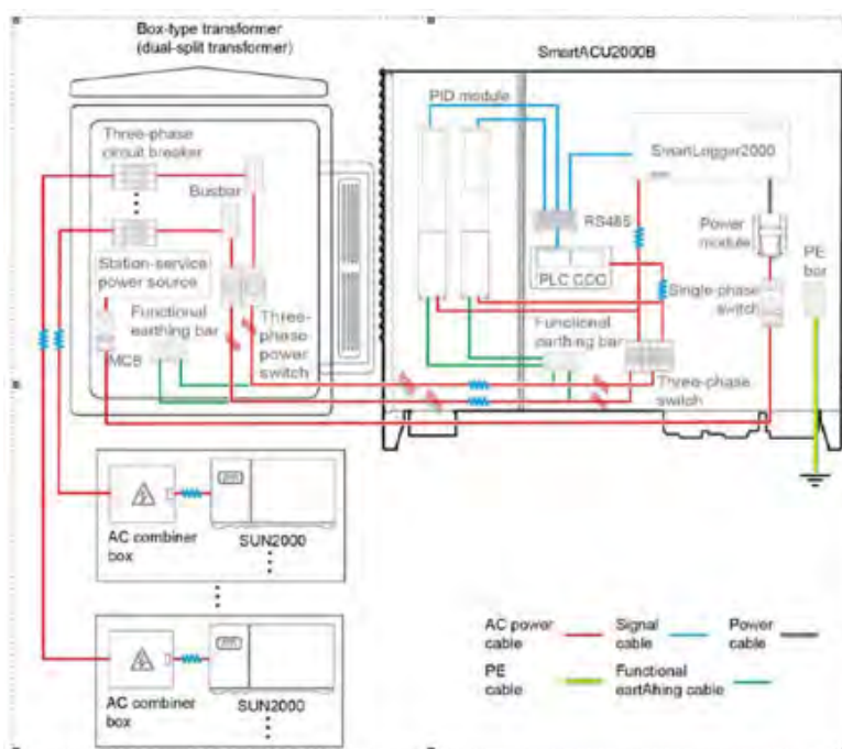
Ilustración 8: Módulo anti-PID
