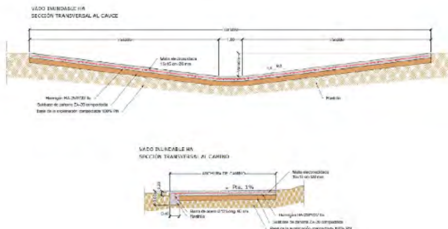
Ilustración 12: Acondicionamiento de vado existente.
