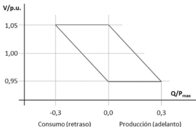
Ilustración 8: Diagrama U-Q/P de un módulo de generación de electricidad síncrono tipo C cuando P_{max} < 15 \text{ MW} .
