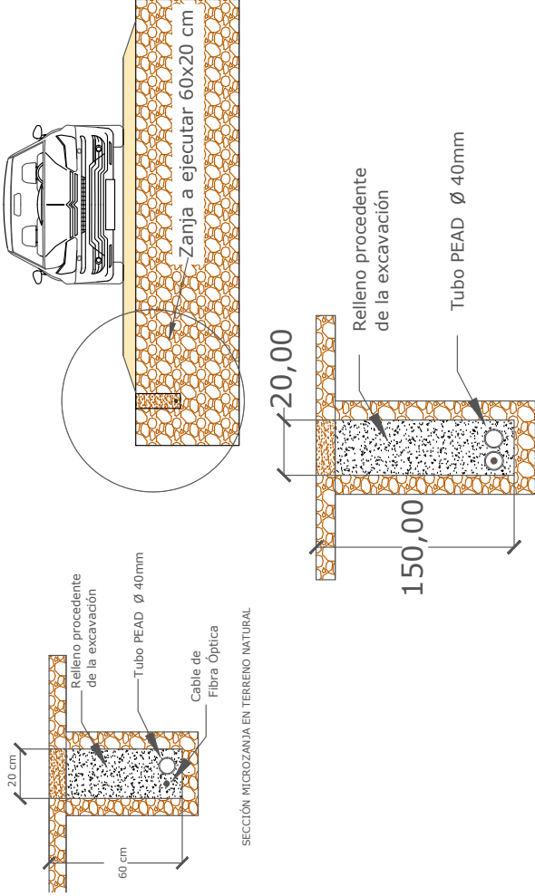
SECCIÓN MICROZANJA EN CUENCA PÚBLICA
