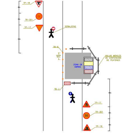
OBRAS OCUPANDO UN CARRIL EN VIAS DE DOS CARRILES. UNO PARA CADA SENTIDO. ORDENACION DEL TRAFICO MEDIANTE SEÑALISTAS.
