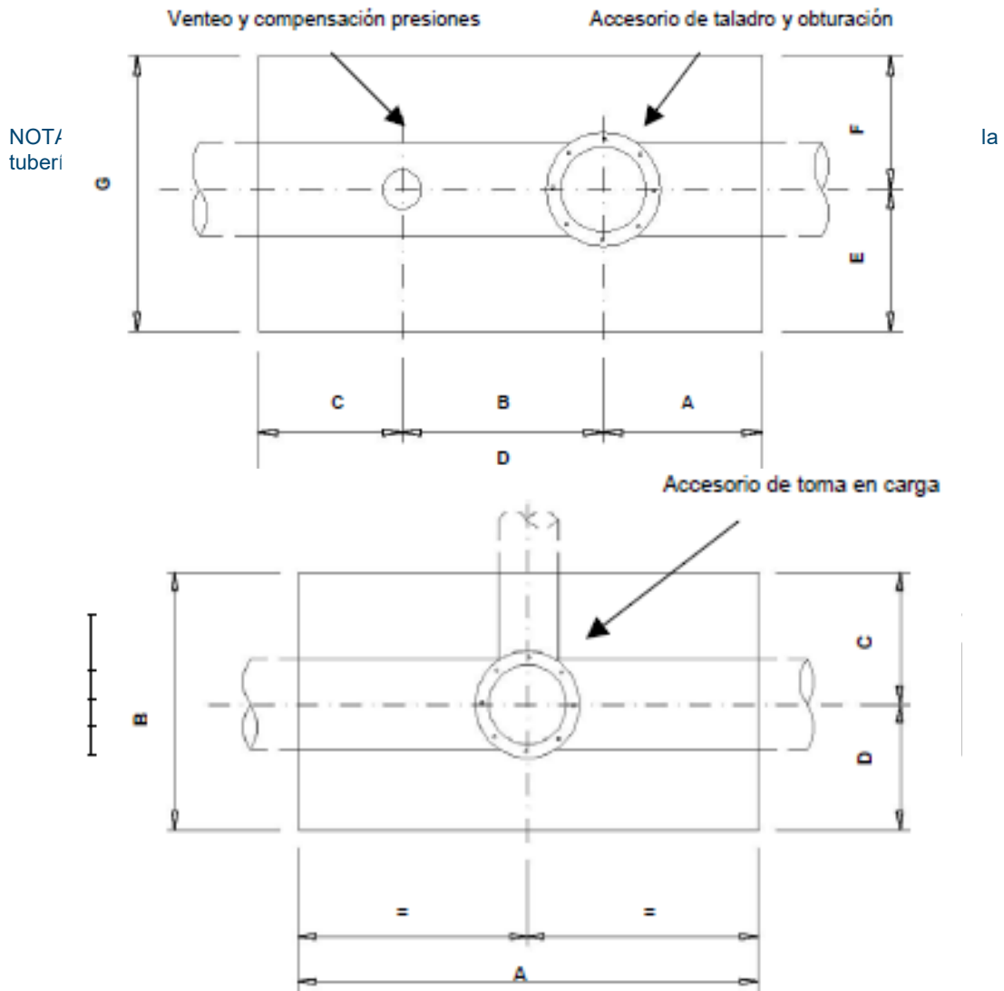
Figura.1-Dimensiones de zanjas en Taladros Simples
