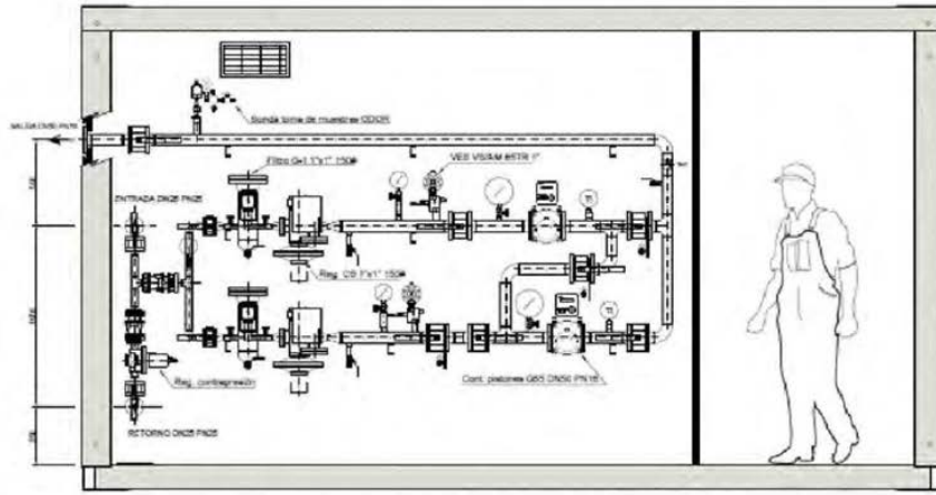
SECCION A-B
