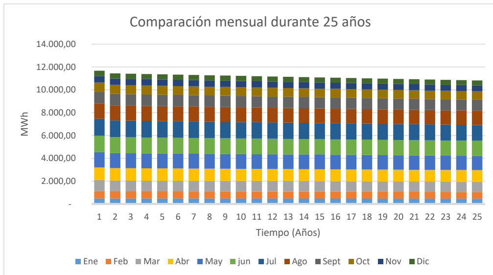
Gráfica 2 - Energía mensual producida durante 25 años
