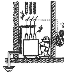
4. Poner a tierra y en cortocircuito.
