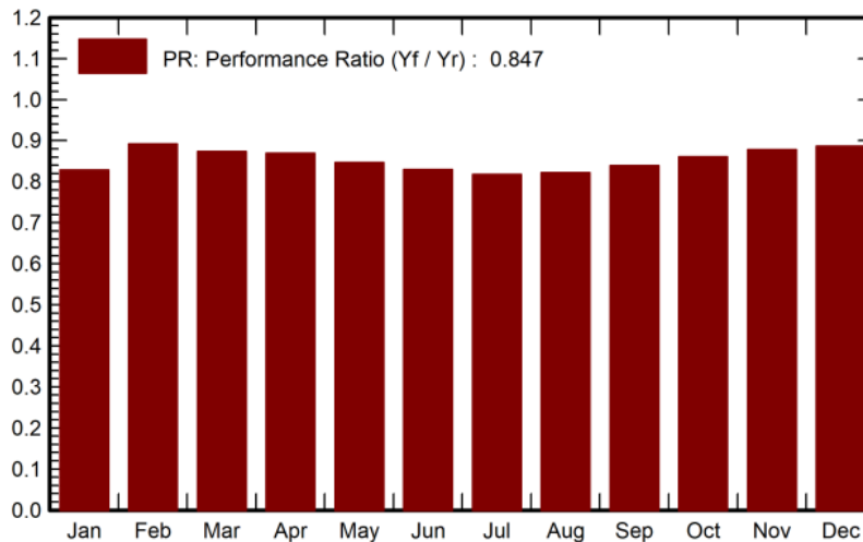
Gráfica 1 - Representación gráfica del Performance Ratio (PR)
