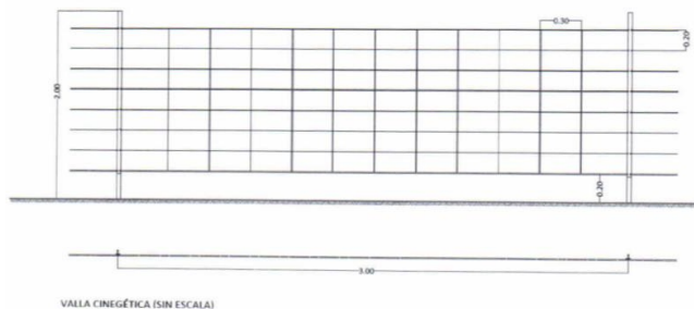
Ilustración 3: Detalle del vallado cinegético
