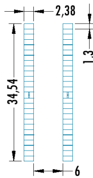
Ilustración 1: Configuración física de los módulos (1V25)
