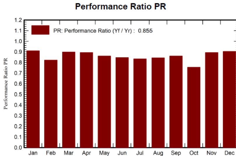
Gráfica 1 - Representación gráfica del Performance Ratio (PR)
