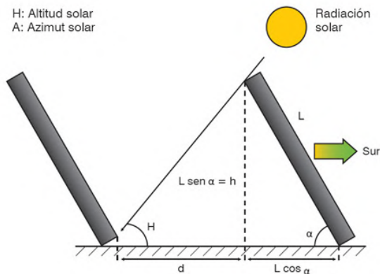
Ilustración 2: Cálculo del pitch
