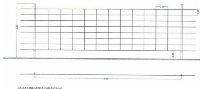
Ilustración 3: Detalle del vallado cinético
