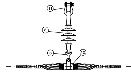
GRAPA ARMADA
