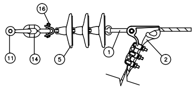
AMARRE SENCILLO CON GRAPA
