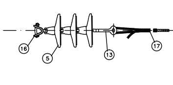
AMARRE SENCILLO CON PERFORMADO
