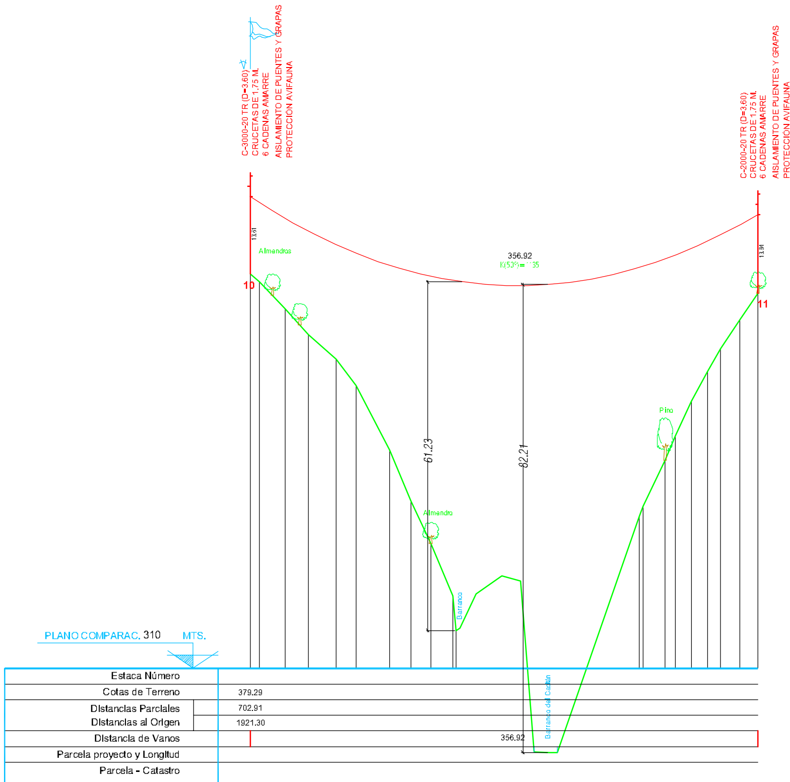
PERFIL
