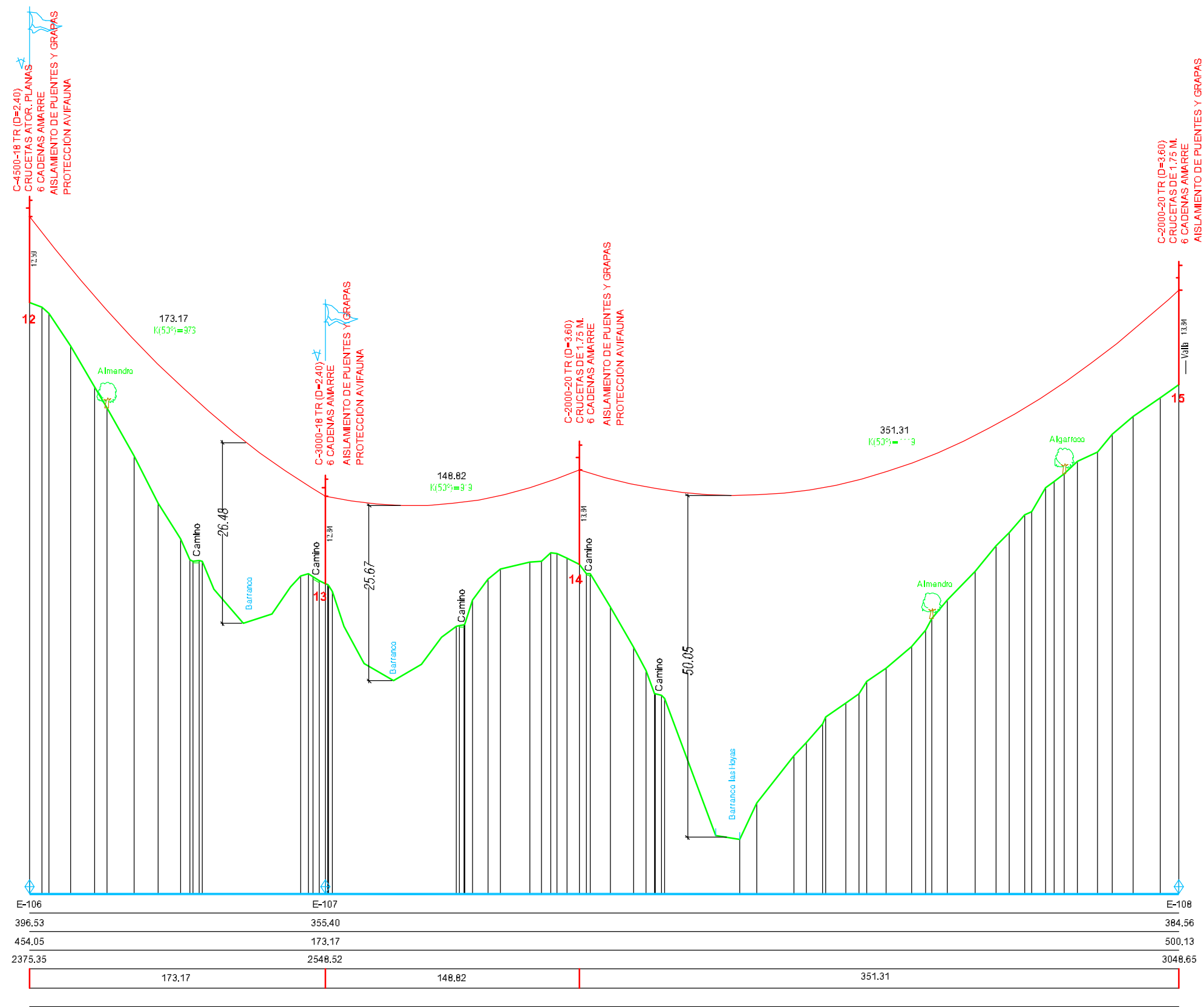
PERFIL
