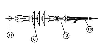
AMARRE SENCILLO CON PERFORMADO
