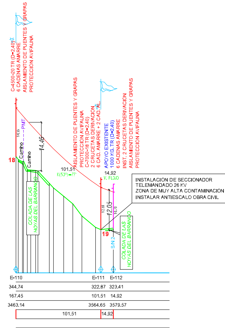
PERFIL
