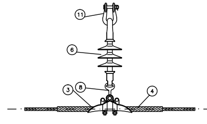
CON PREFORMADO (ARMOR ROD)
