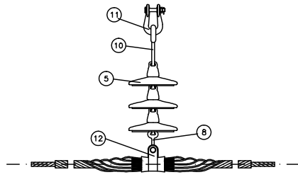
GRAPA ARMADA
