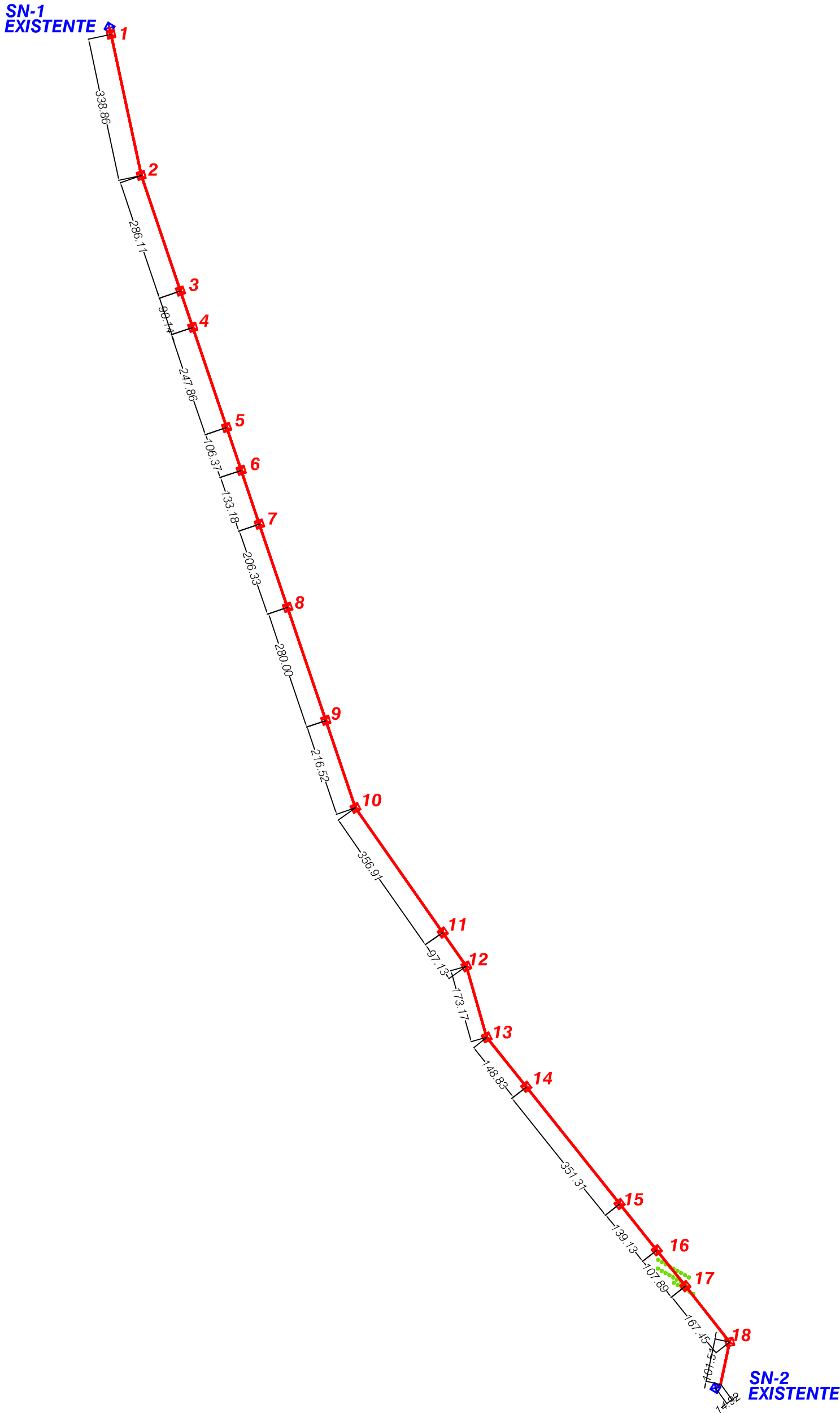
ESQUEMA UNIFILAR DE NUEVO CIERRE DE LÍNEAS (20 KV) "CHERIN" (SU. ALCOLEA) Y "LIMITE_PRO" (SUB.BERJA) CONDUCTOR LARL 125 E
