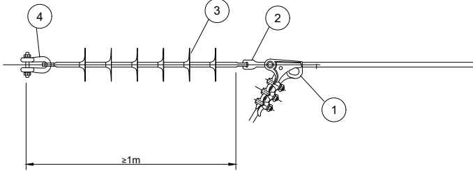
AISLADOR POLIMÉRICO PARA AMARRE
