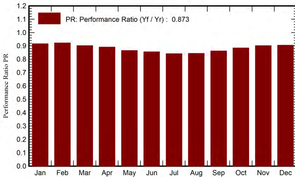
Gráfica 1 - Representación gráfica del Performance Ratio (PR)
