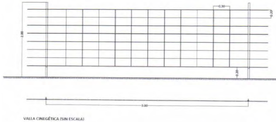
Ilustración 3: Detalle del vallado cinegético
