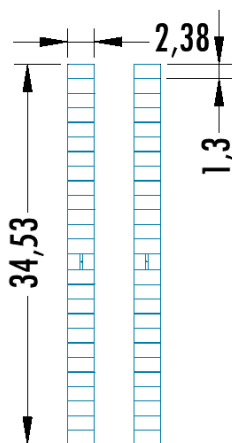
Ilustración 1: Configuración física de los módulos (1V25)
