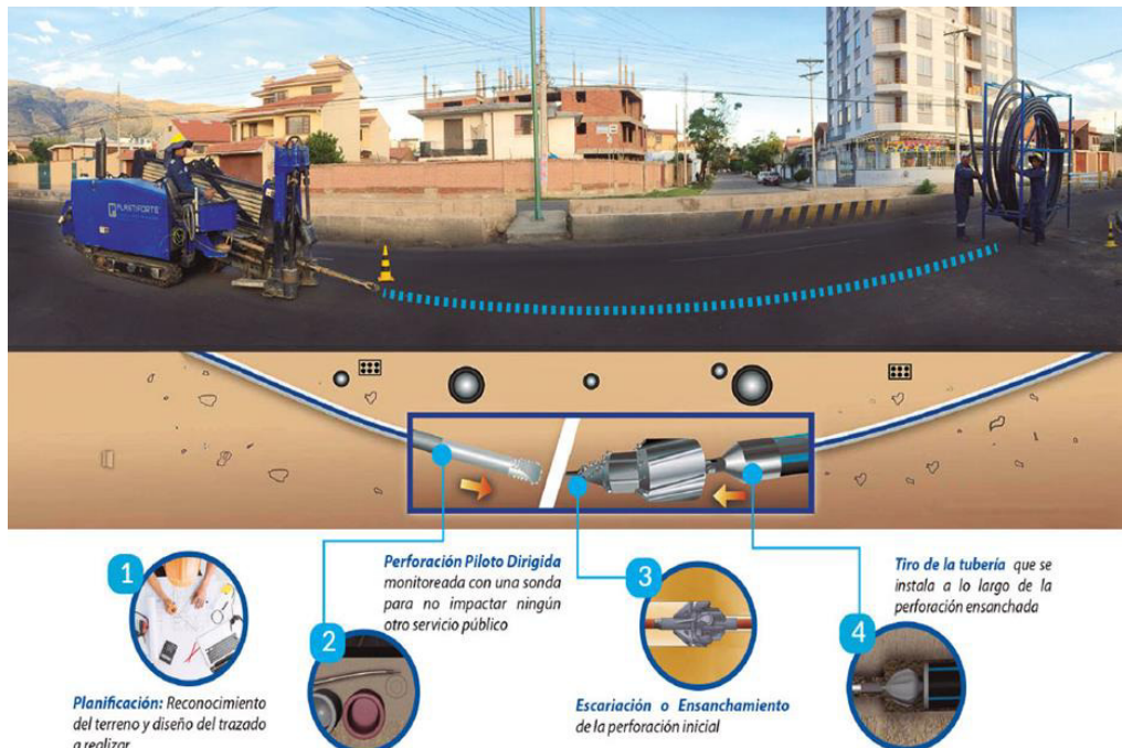
Ilustración 4- Perforación dirigida
