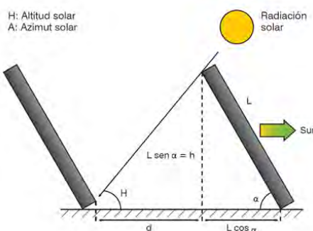
Ilustración 2: Cálculo del pitch
