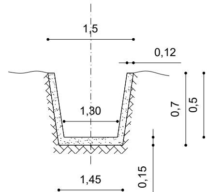
Sección Transversal del Canal a emballar
