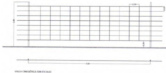
Ilustración 3: Detalle del vallado cinegético
